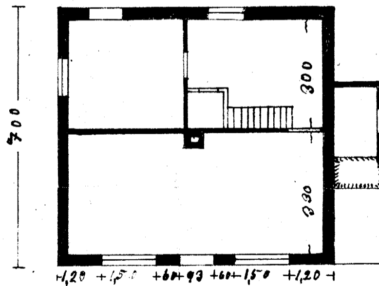
KIALLARI
