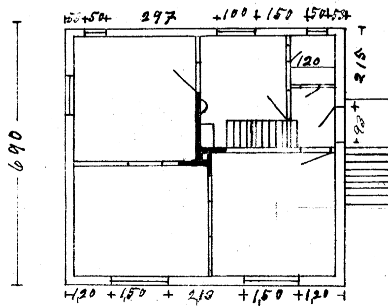
HÆÐ
