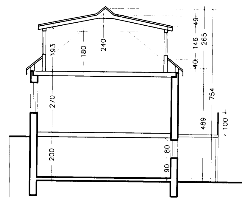
Sneiðing 1:100
