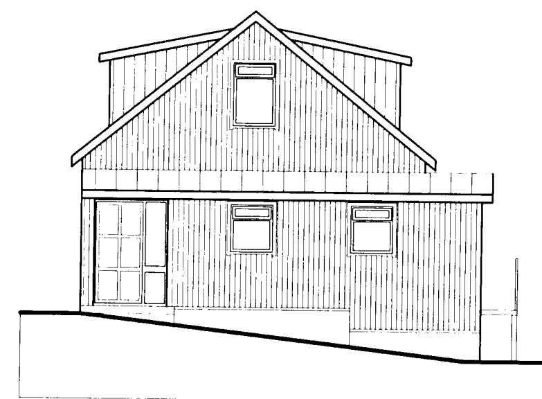
Útlit Norðaustur 1:100
