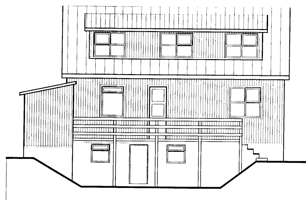
Útlit Norðvestur 1:100
