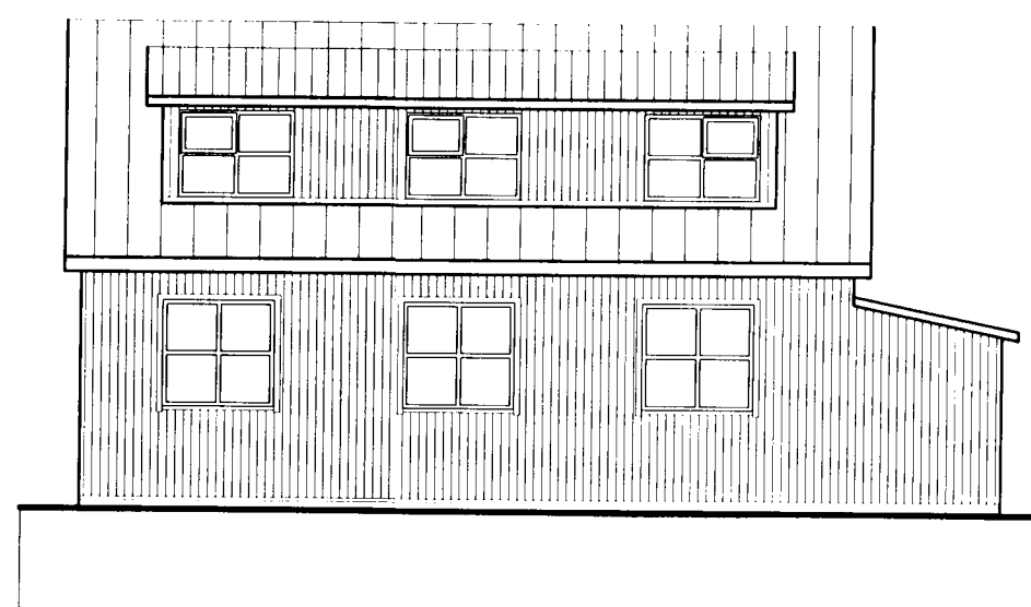
Útlit Suðaustur 1:100
