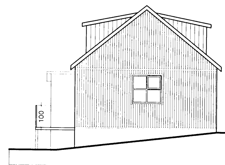
Útlit Suðvestur 1:100
