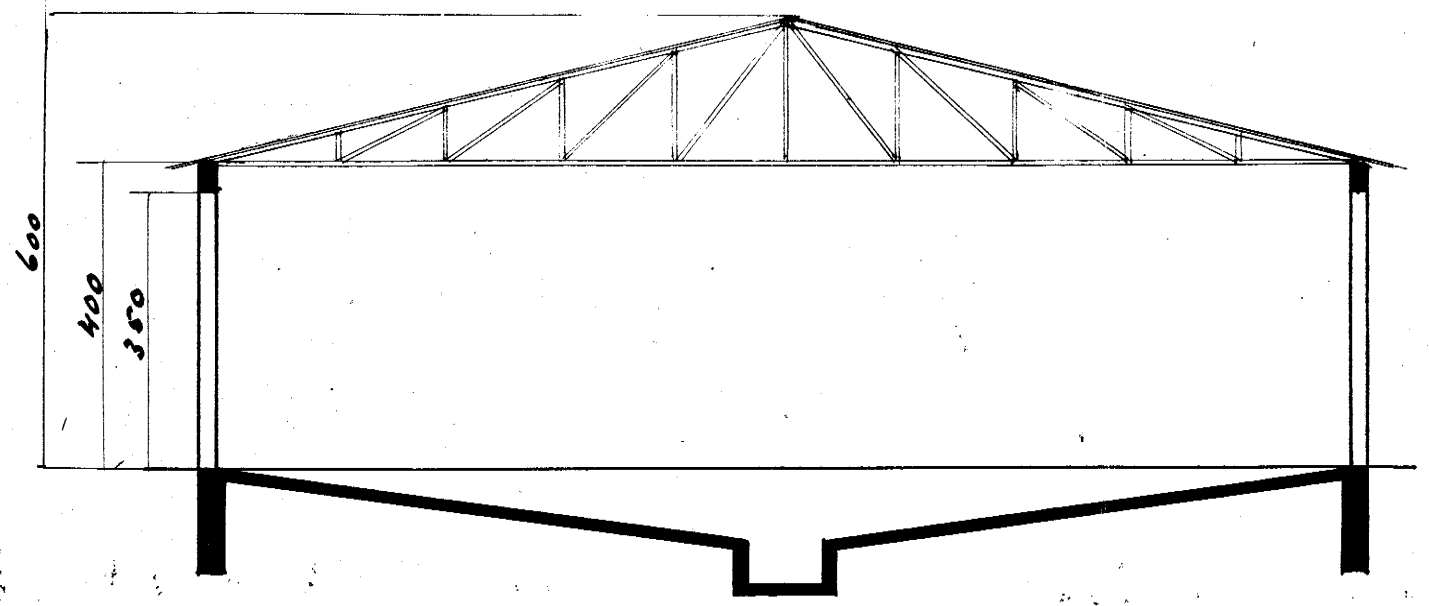
þversk. fiskmottaka
