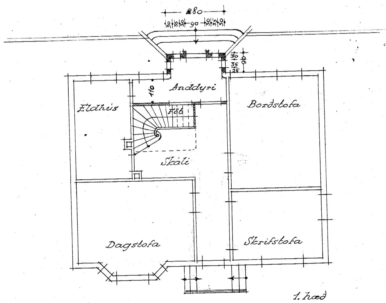
Vesturhlíð
