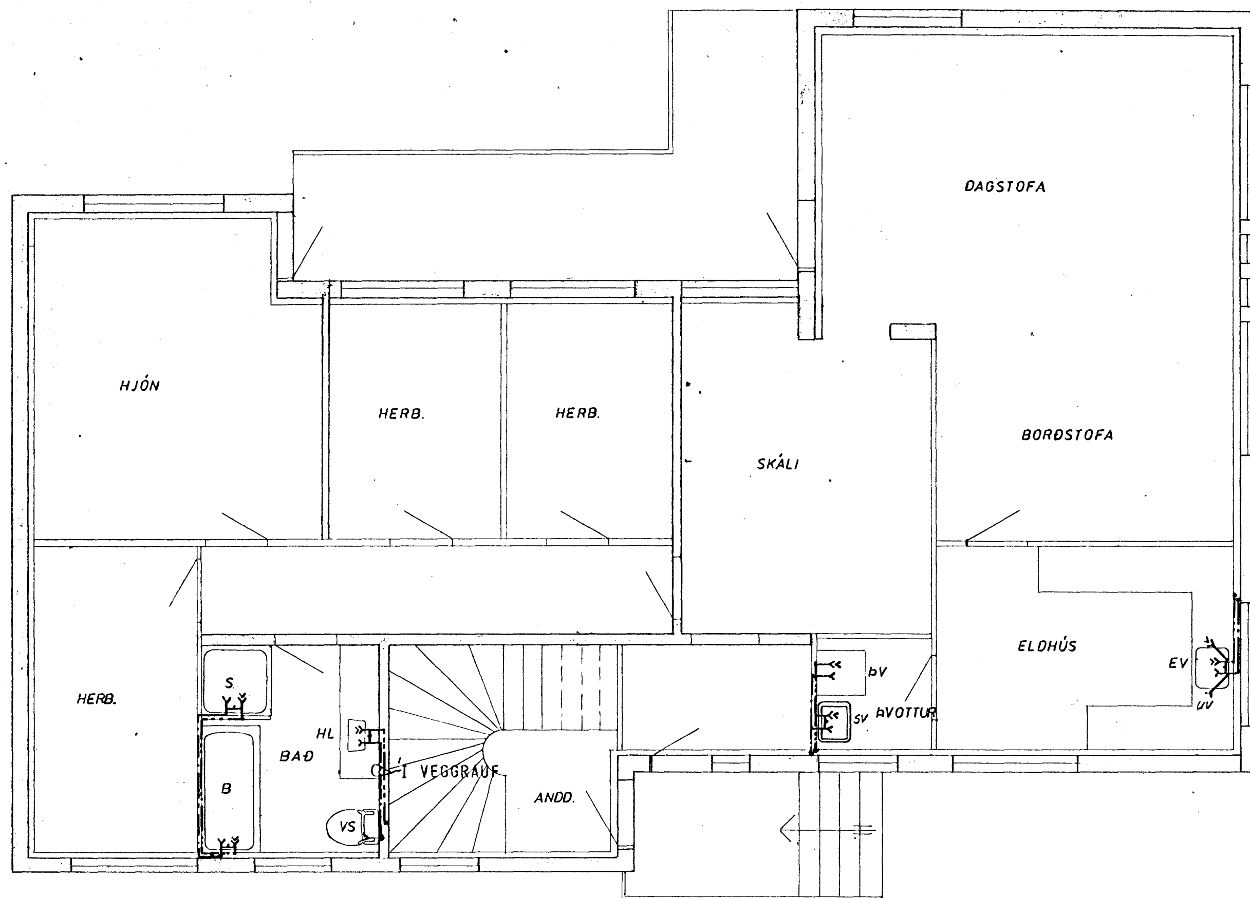
GRUNNMYND HÆÐAR 1:50
