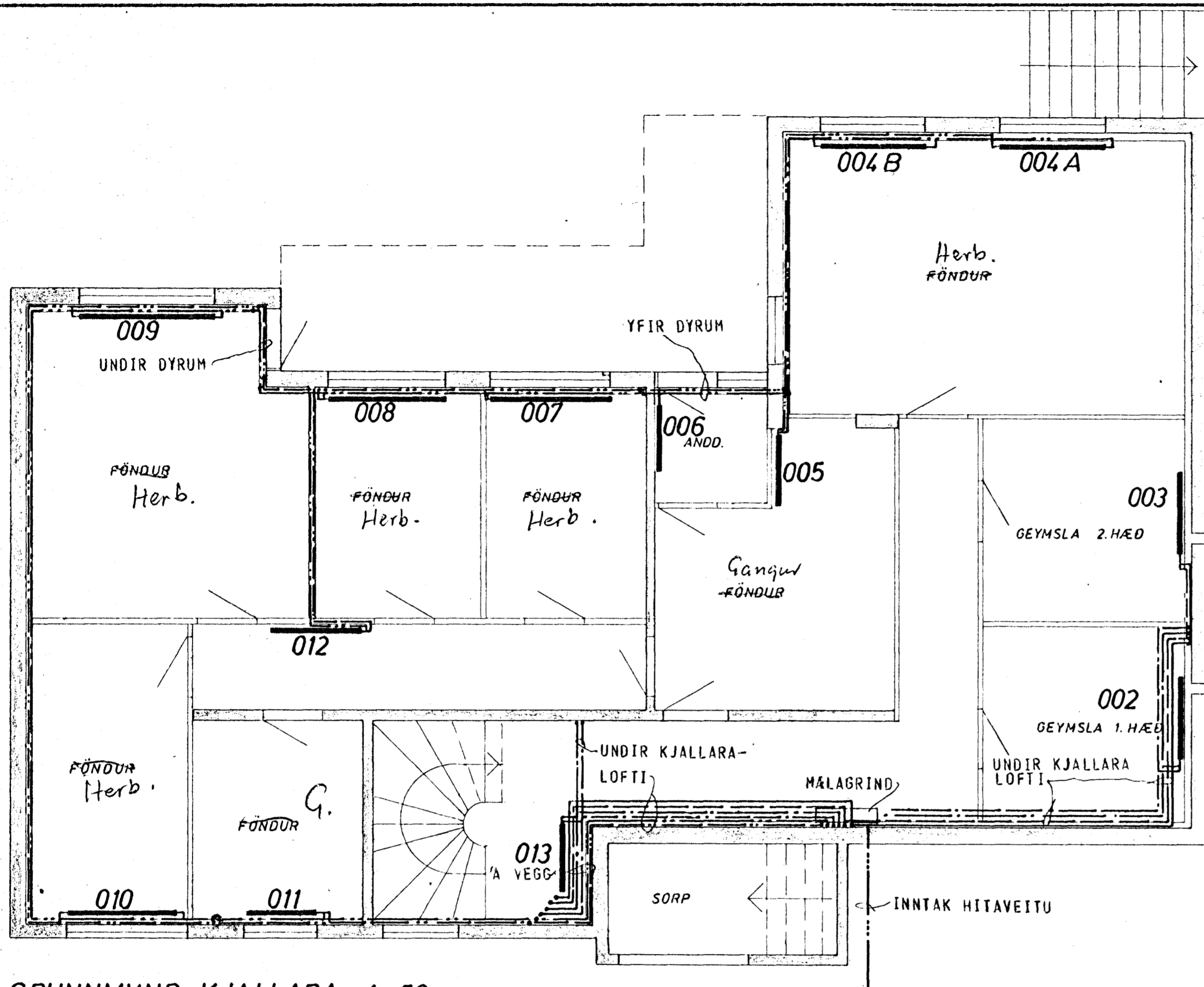
GRUNNMYND KJALLARA 1:50
