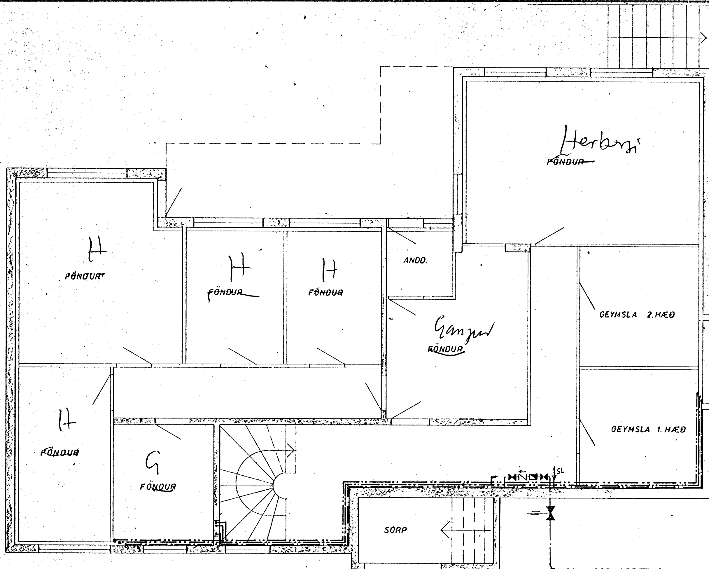
GRUNNMYND KJALLARA 1:50
