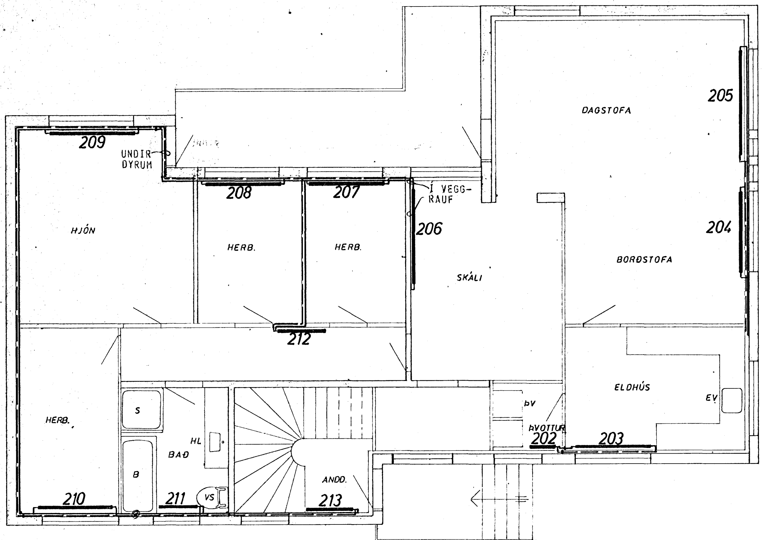
GRUNNMYND HÆÐAR 1:50
