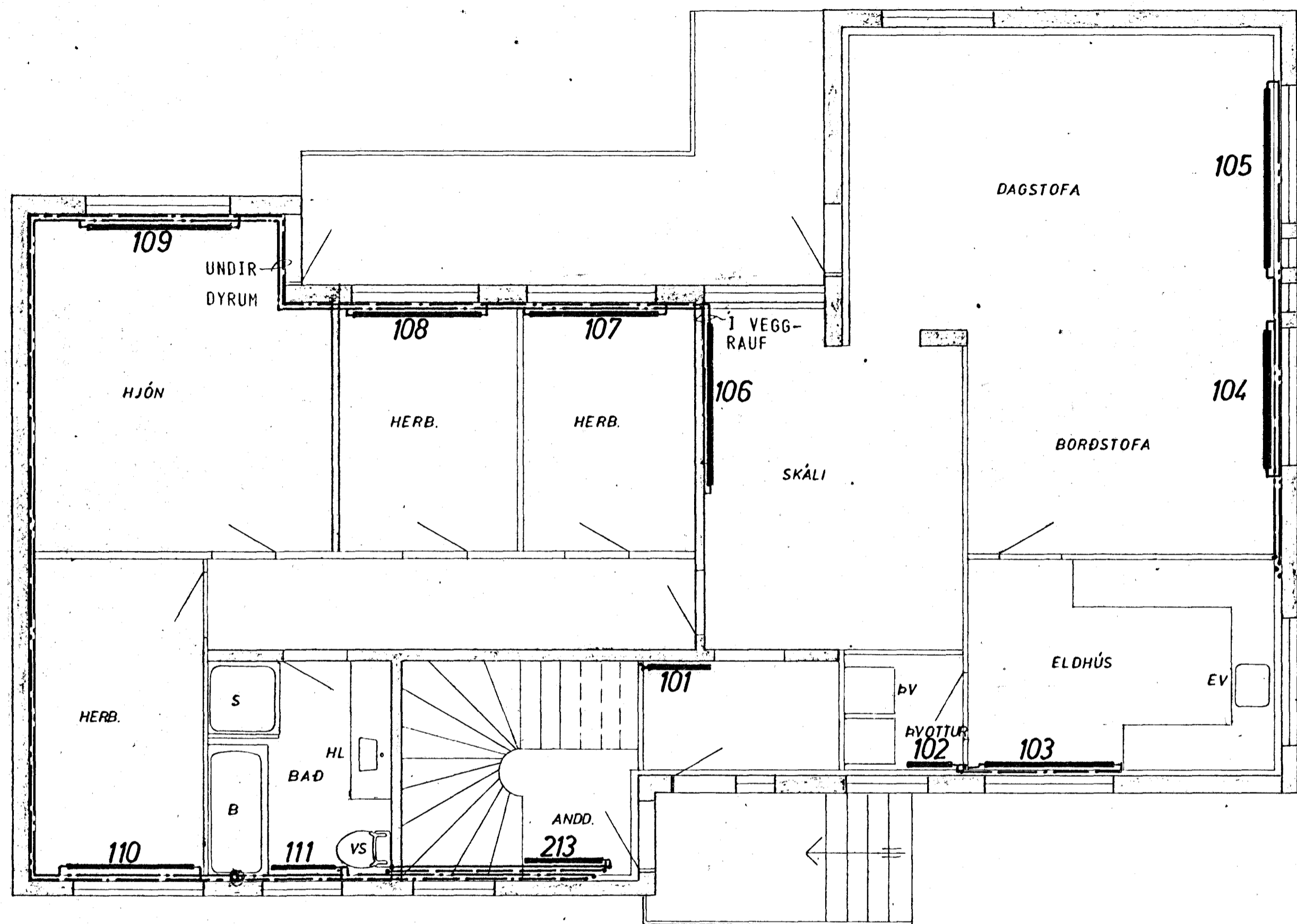
GRUNNMYND HÆÐAR 1:50
