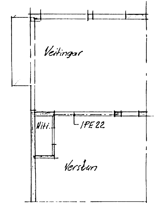
Grunnmynd 1:100
