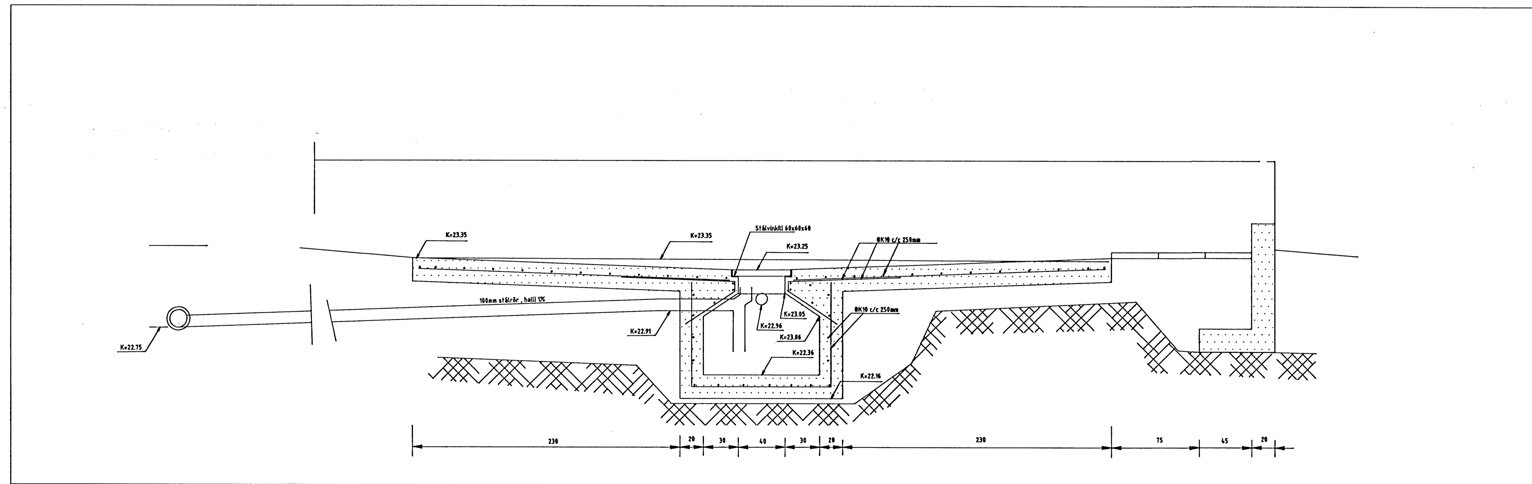
Snið B-B, 1:20
