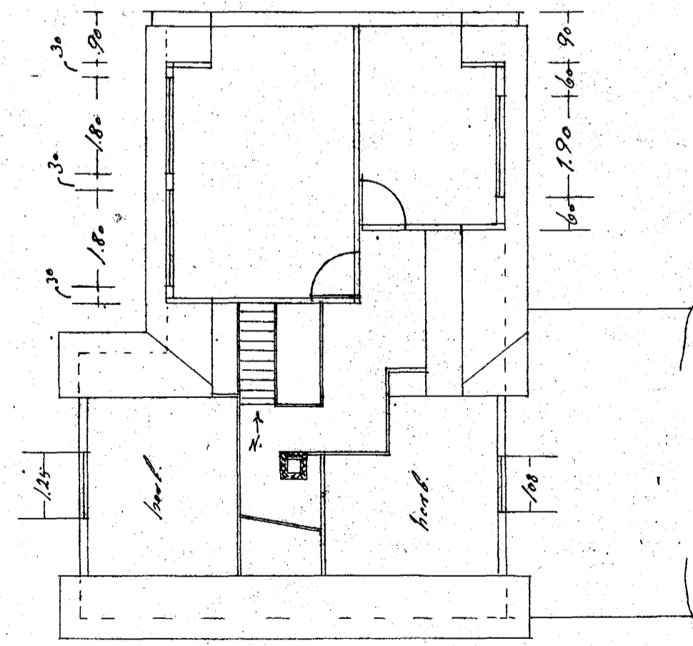
2. hæð
