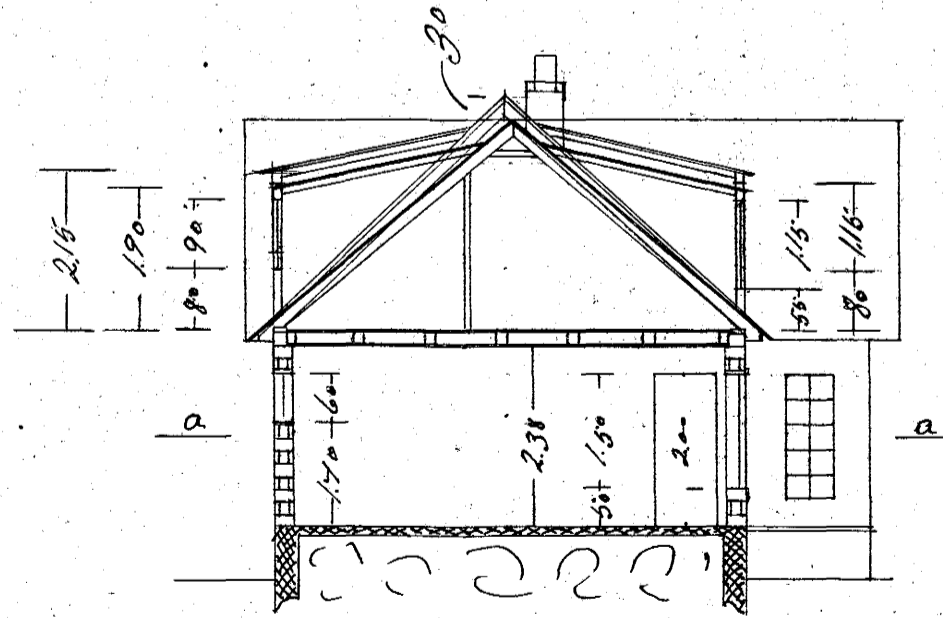
Þverskurður
