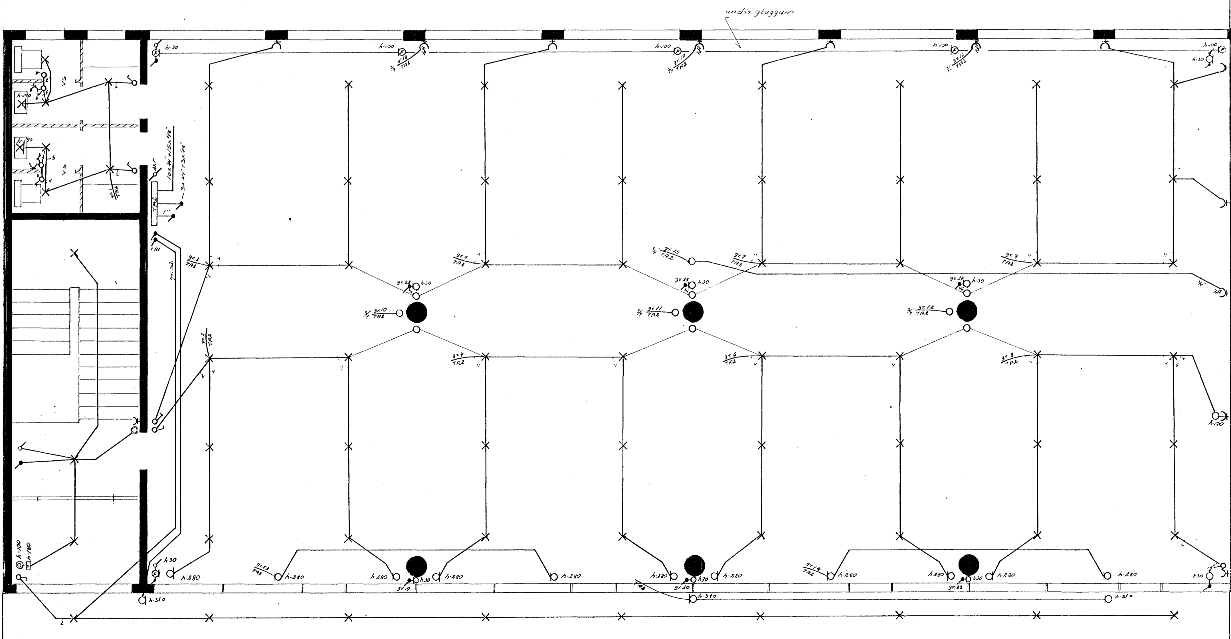
1. hæð
