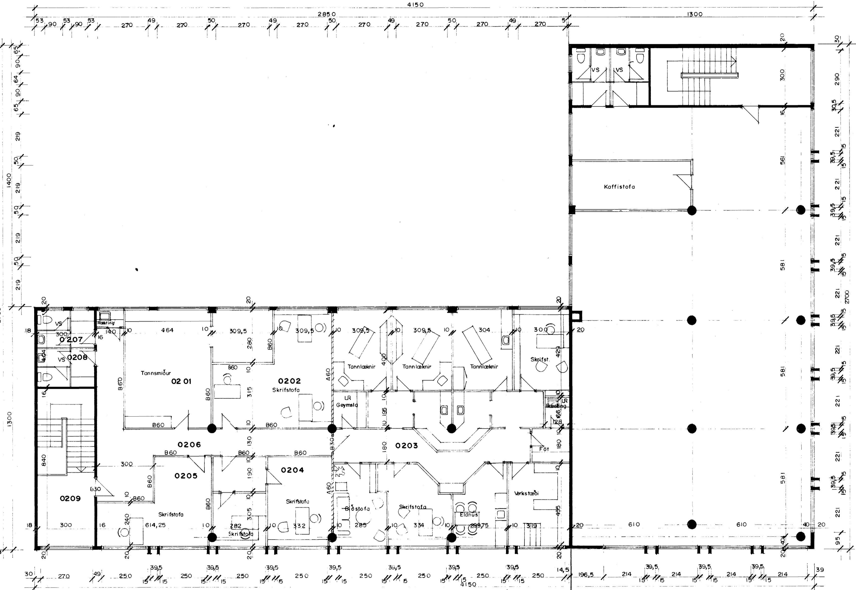
GRUNNMYND 2. HÆÐ
