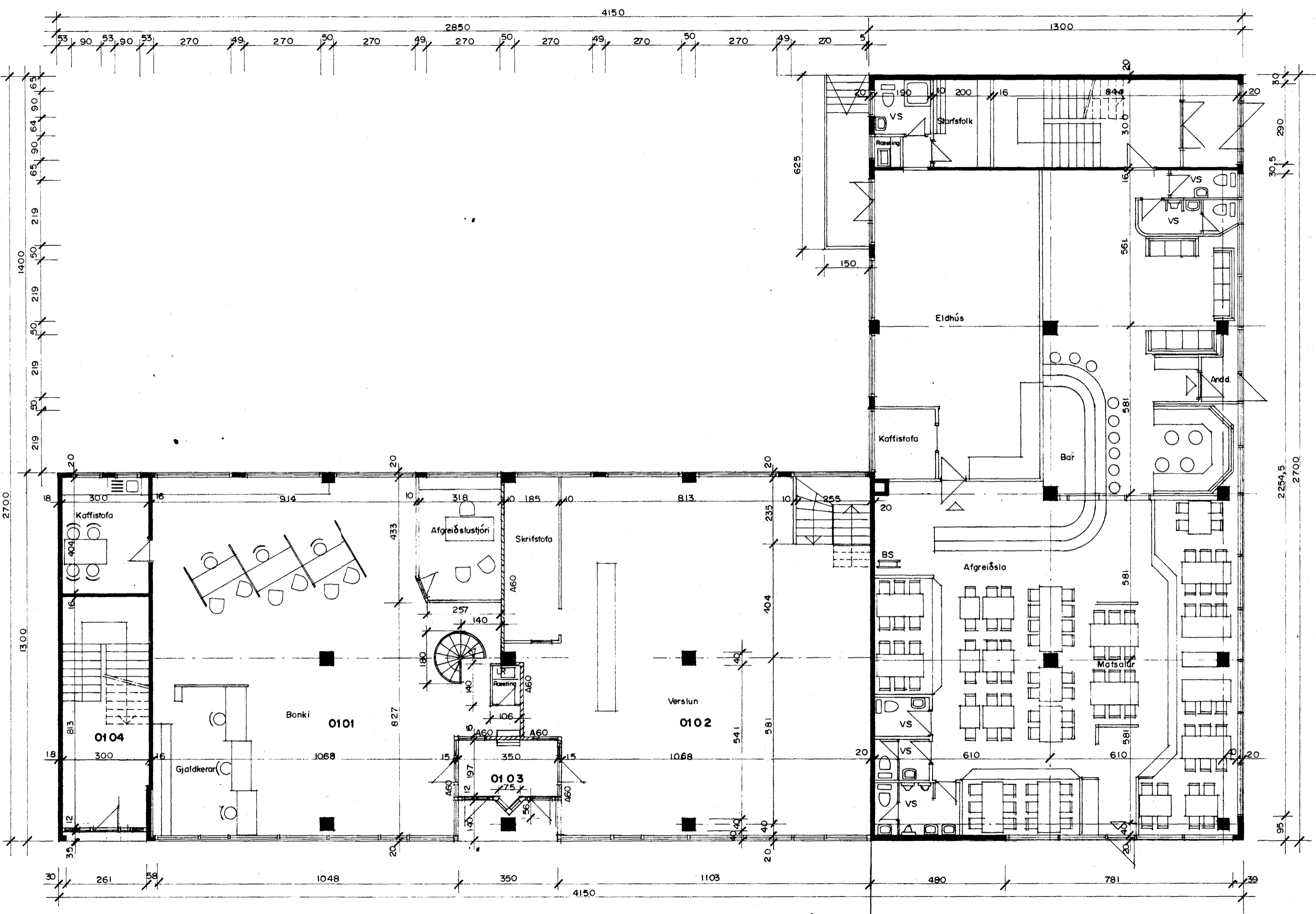
GRUNNMYND 1. HÆÐ
