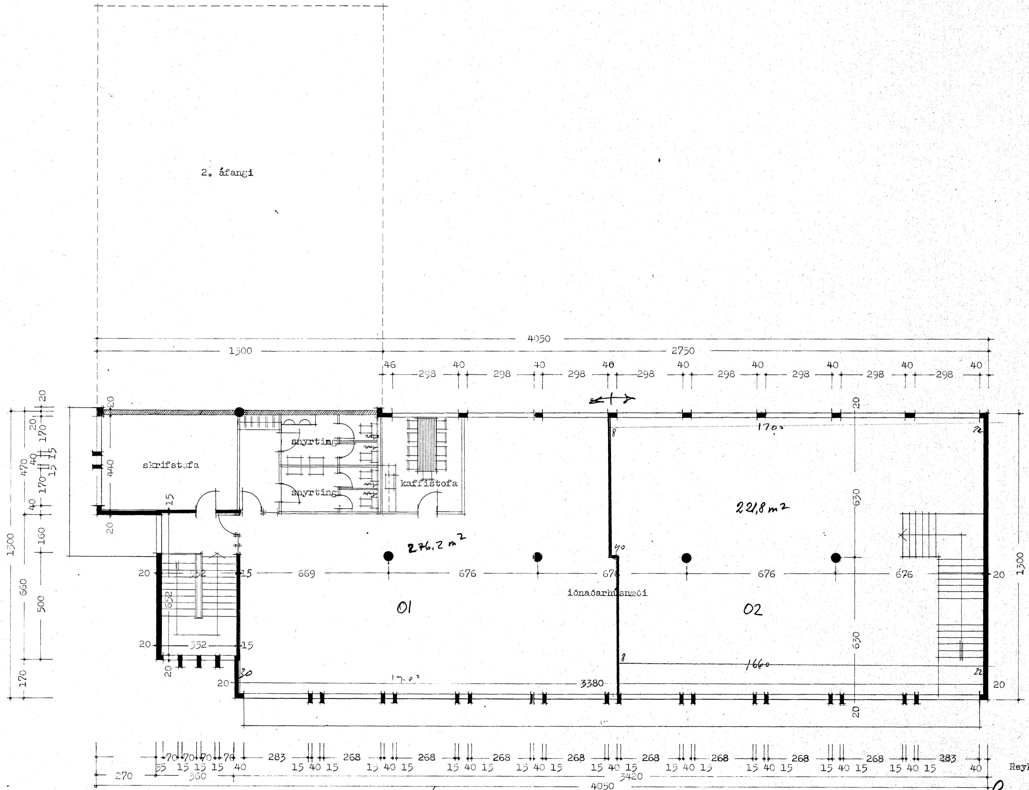
grunnmynd 2. hæð 02
