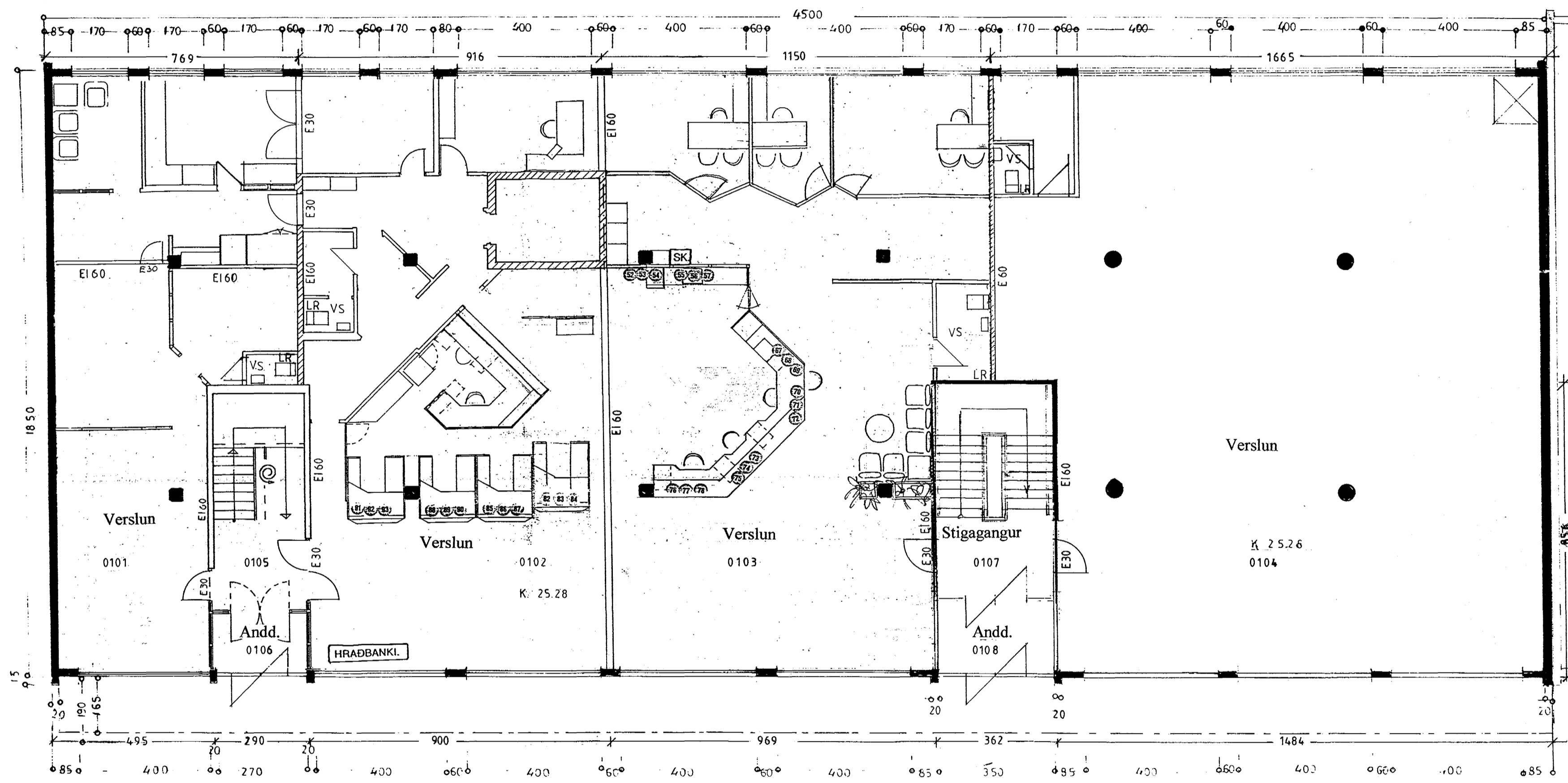
1. Hæð 1/100
