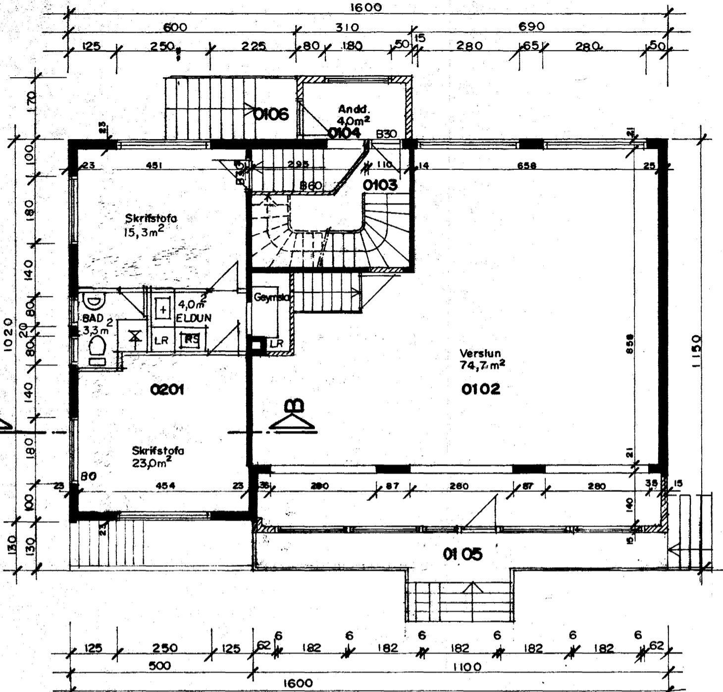
GRUNNMYND 2. HÆÐ
