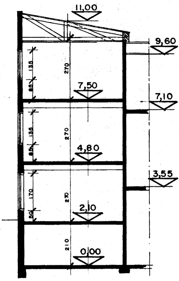
SKURÐUR B-B
