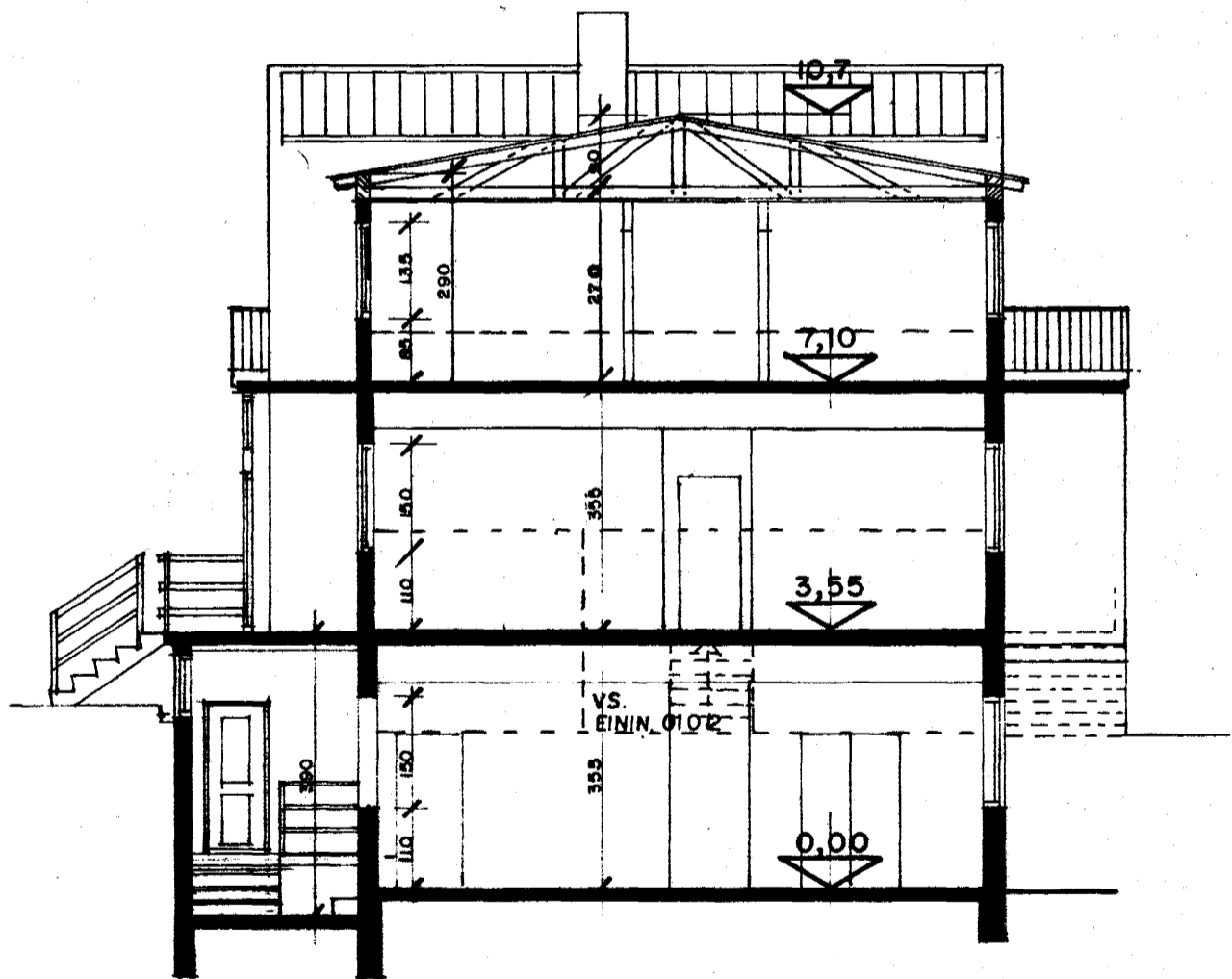
SKURÐUR A-A
