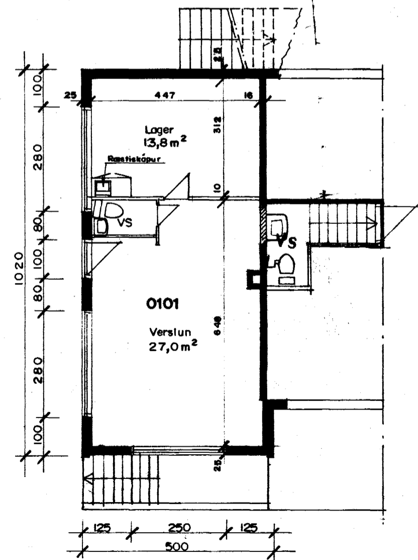
GRUNNMYND 1. HÆÐ
