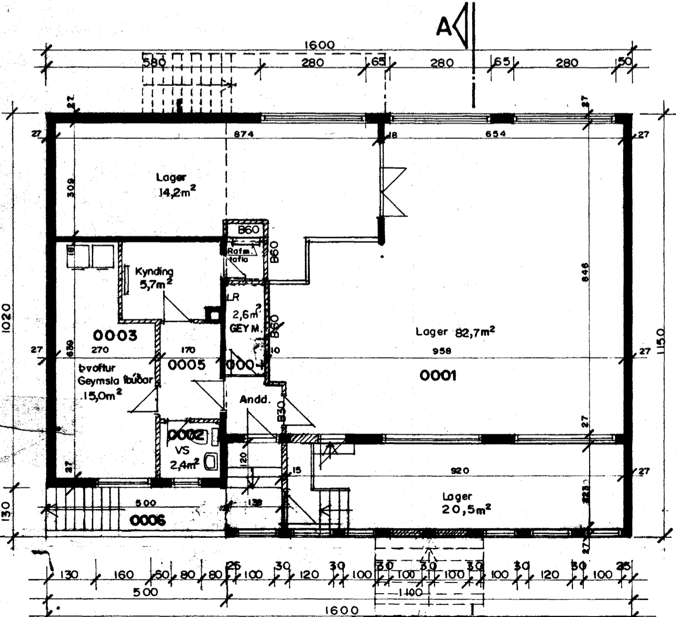
GRUNNMYND KJALLARI
