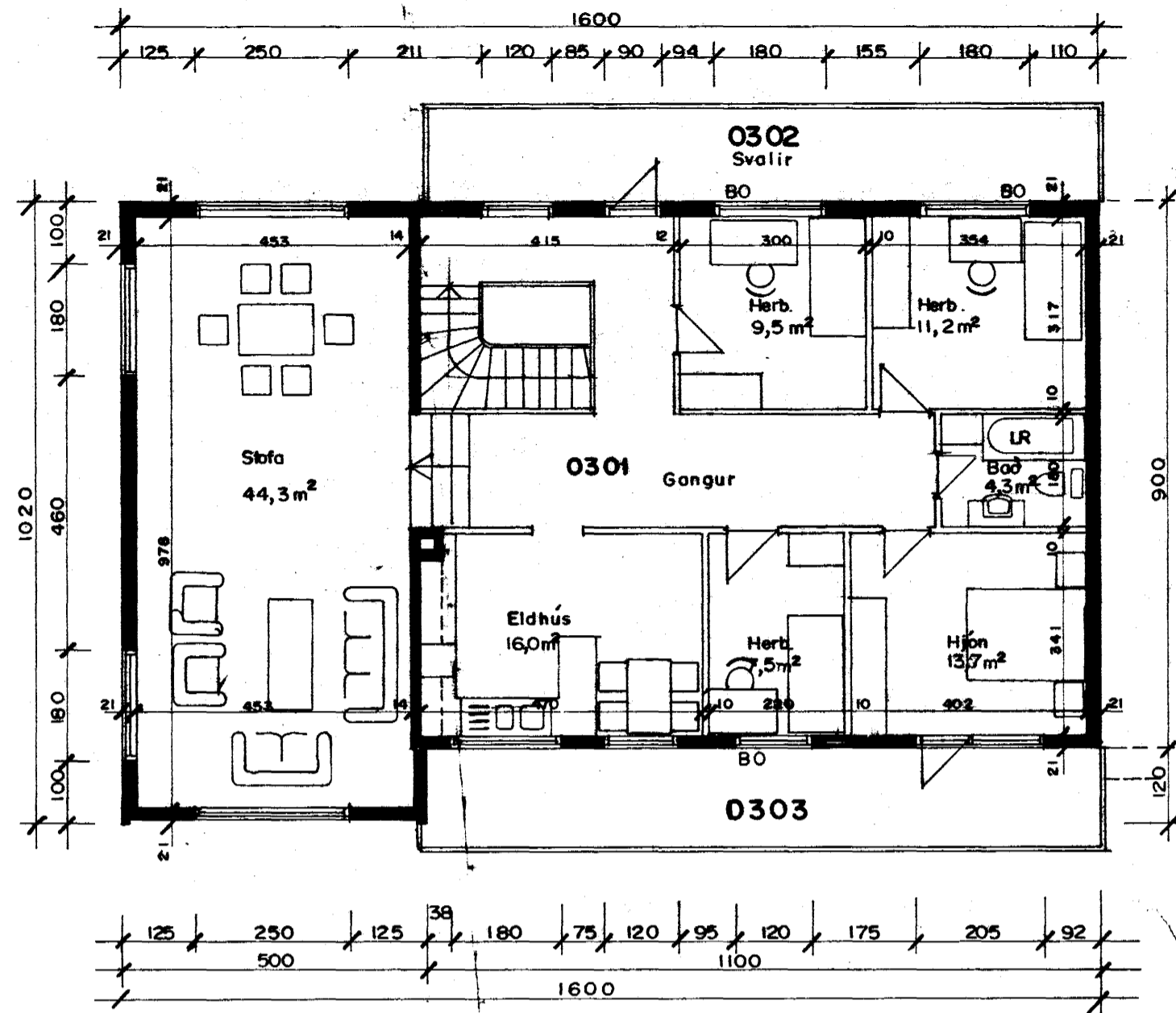
GRUNNMYND 3. HÆÐ
