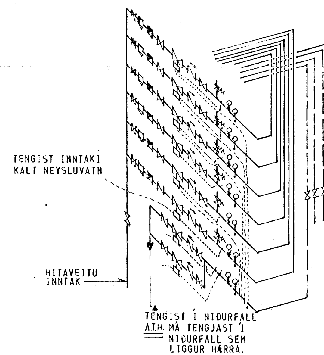
TENGIMYND HITAVEITU 1:20
