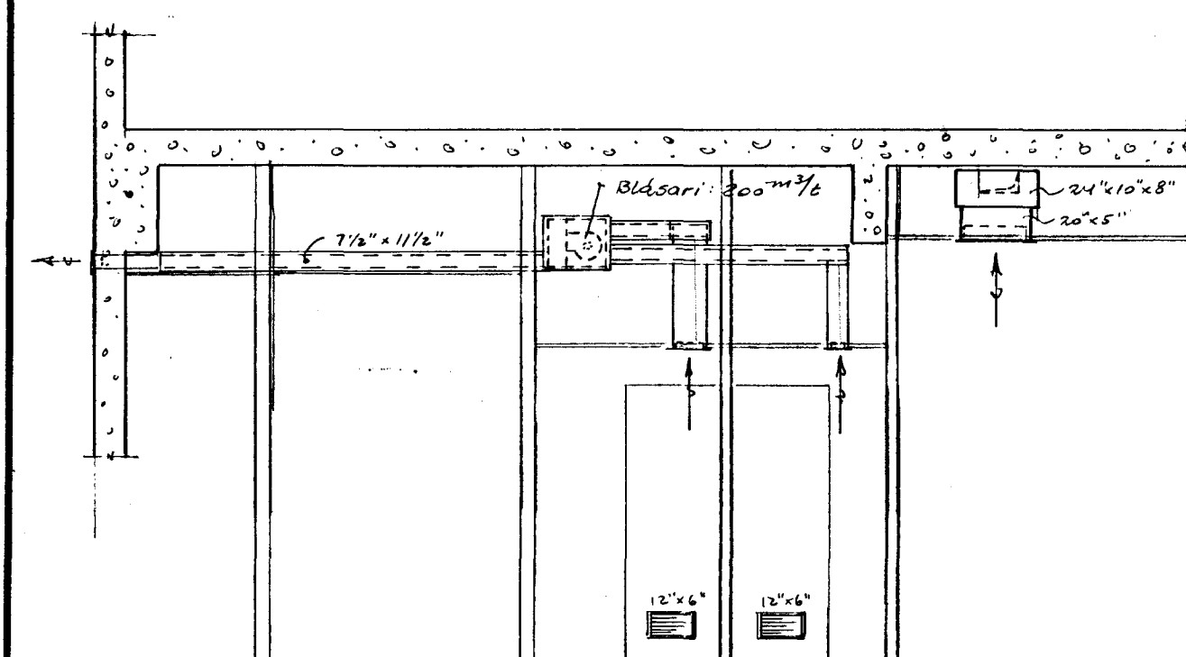
SNID A-A MKV ~ 1:50
