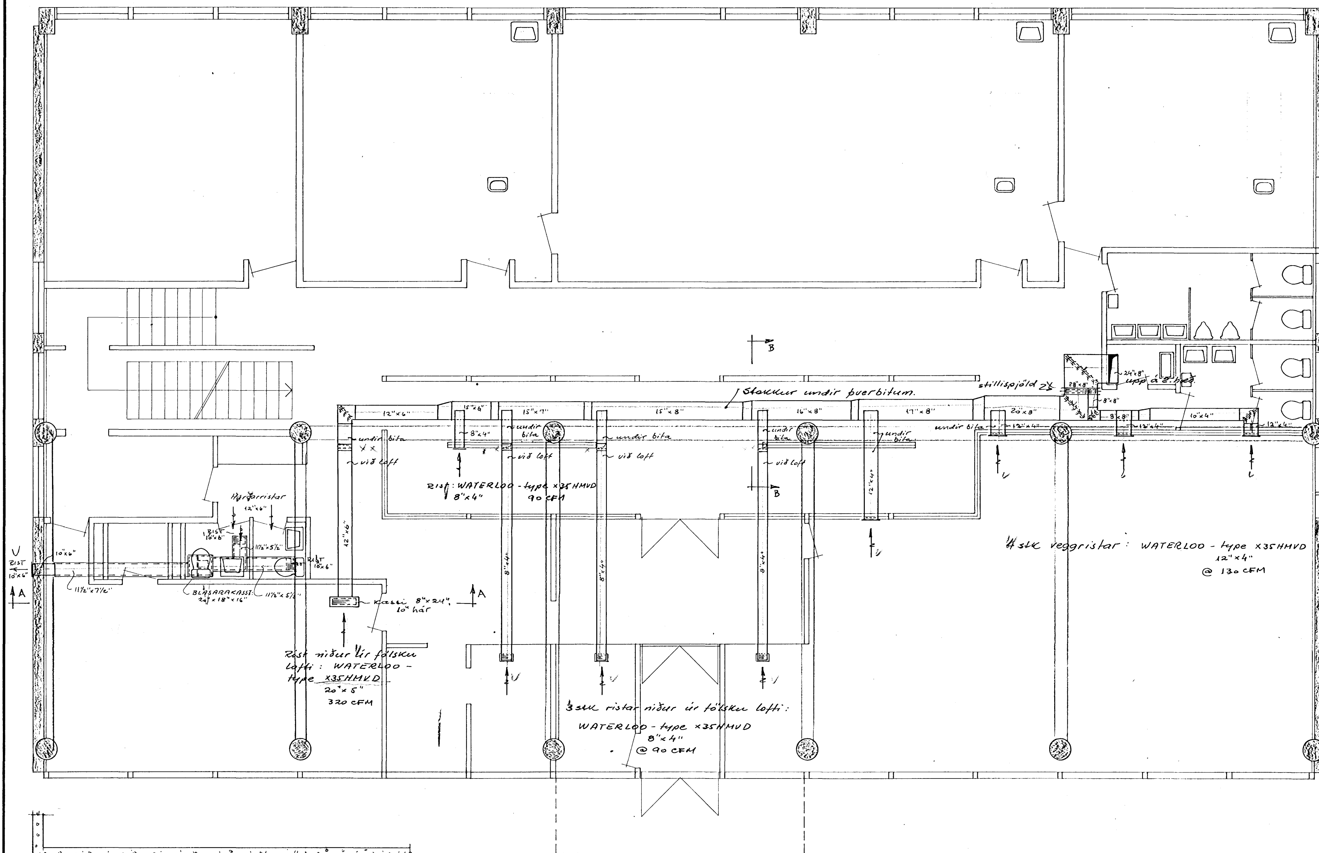
1. HÆÐ
