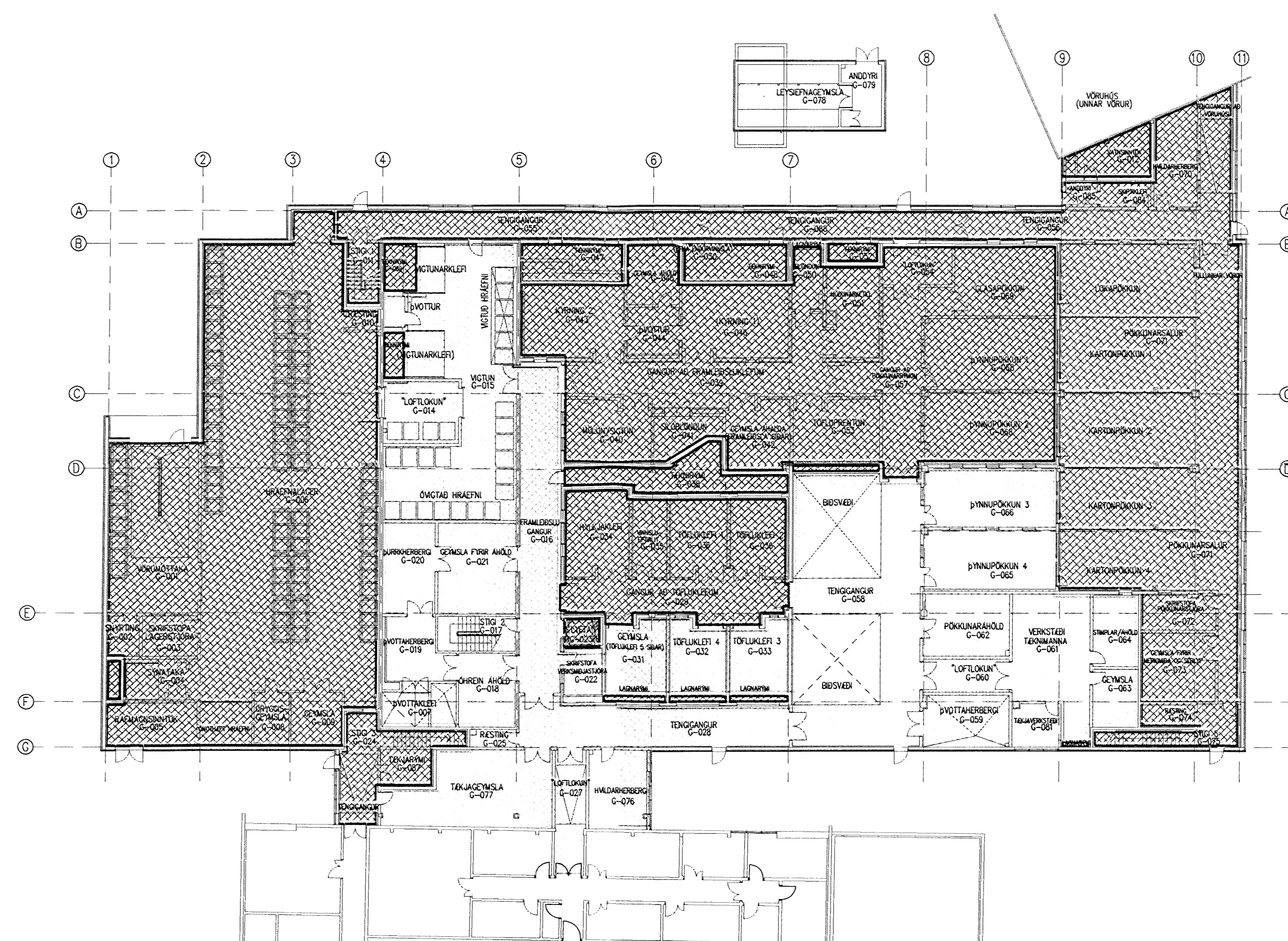
GRUNNMYND NEDRI HÆÐAR.
