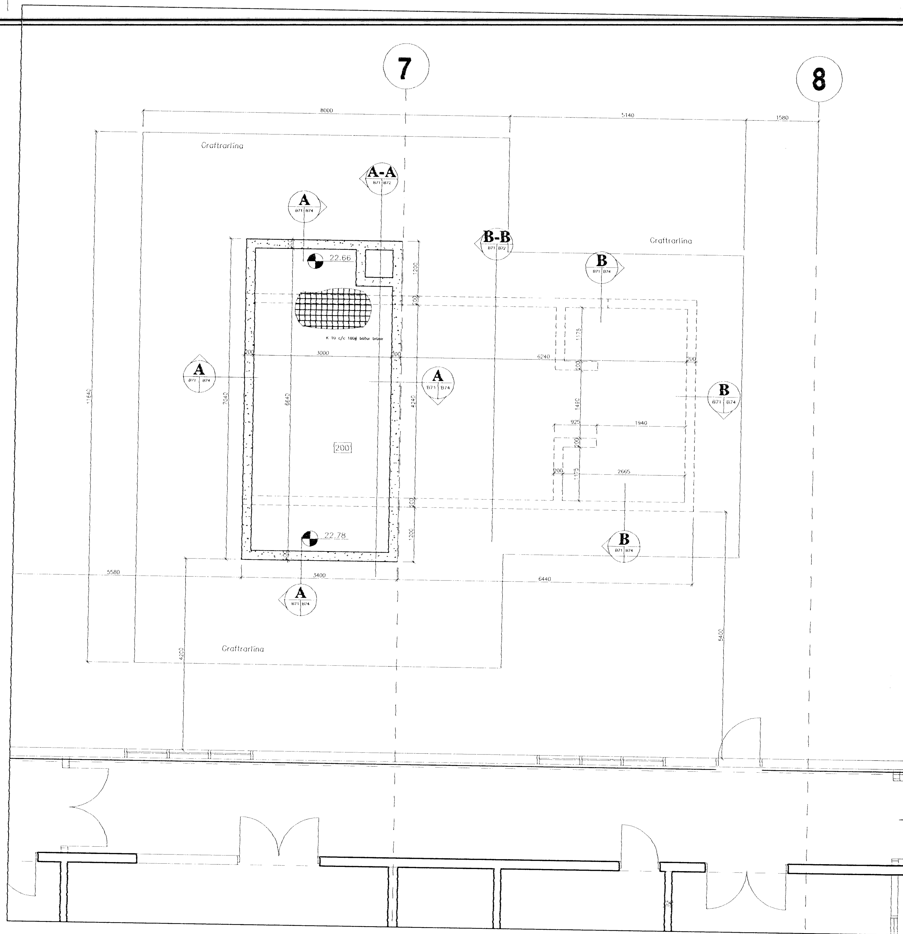
SNID A - A Planmynd sökklar settankur M 1:50
