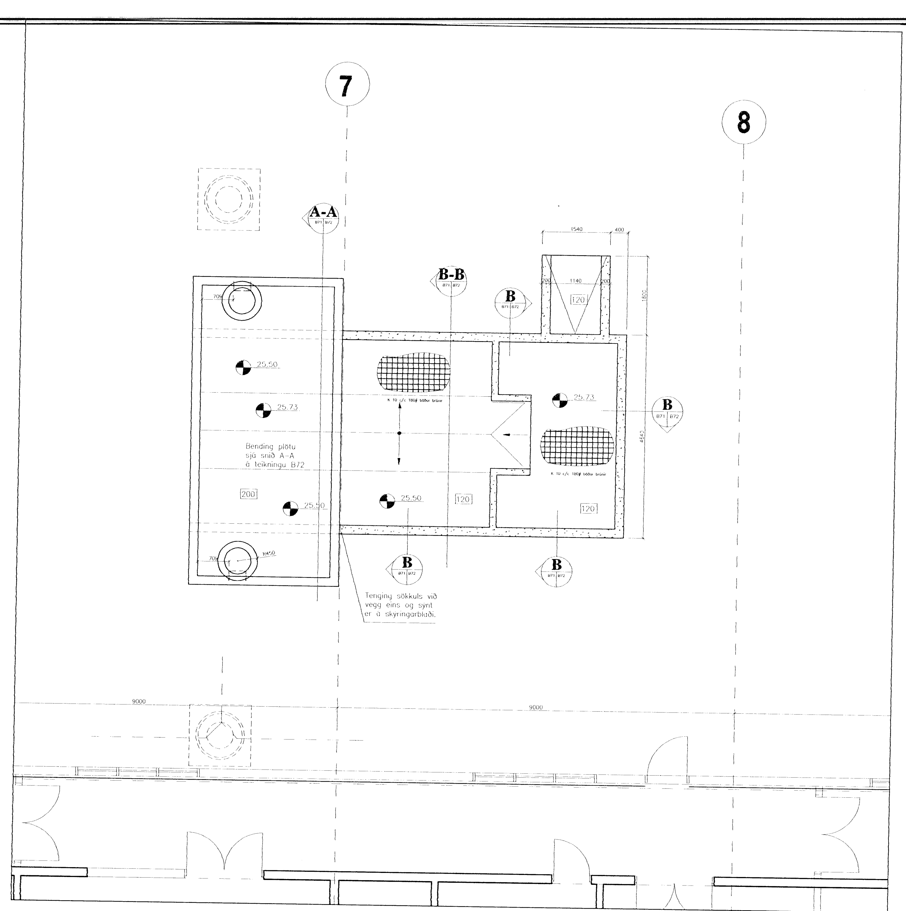
SNID B - B Planmynd sökklar leysiefnageymsla M 1:50
