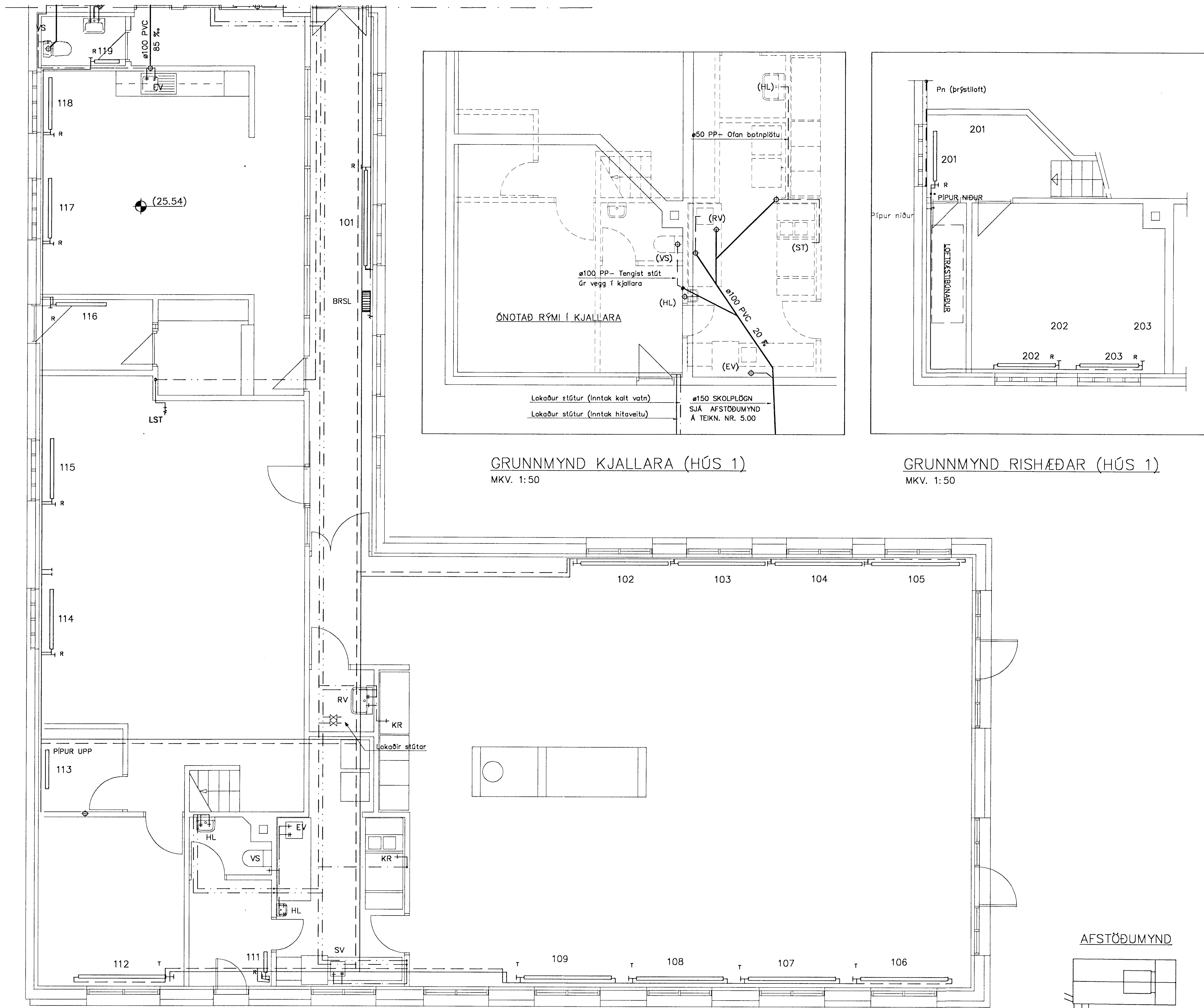
GRUNNMYND 1. HÆÐAR (HÚS 1) MKV. 1:50
