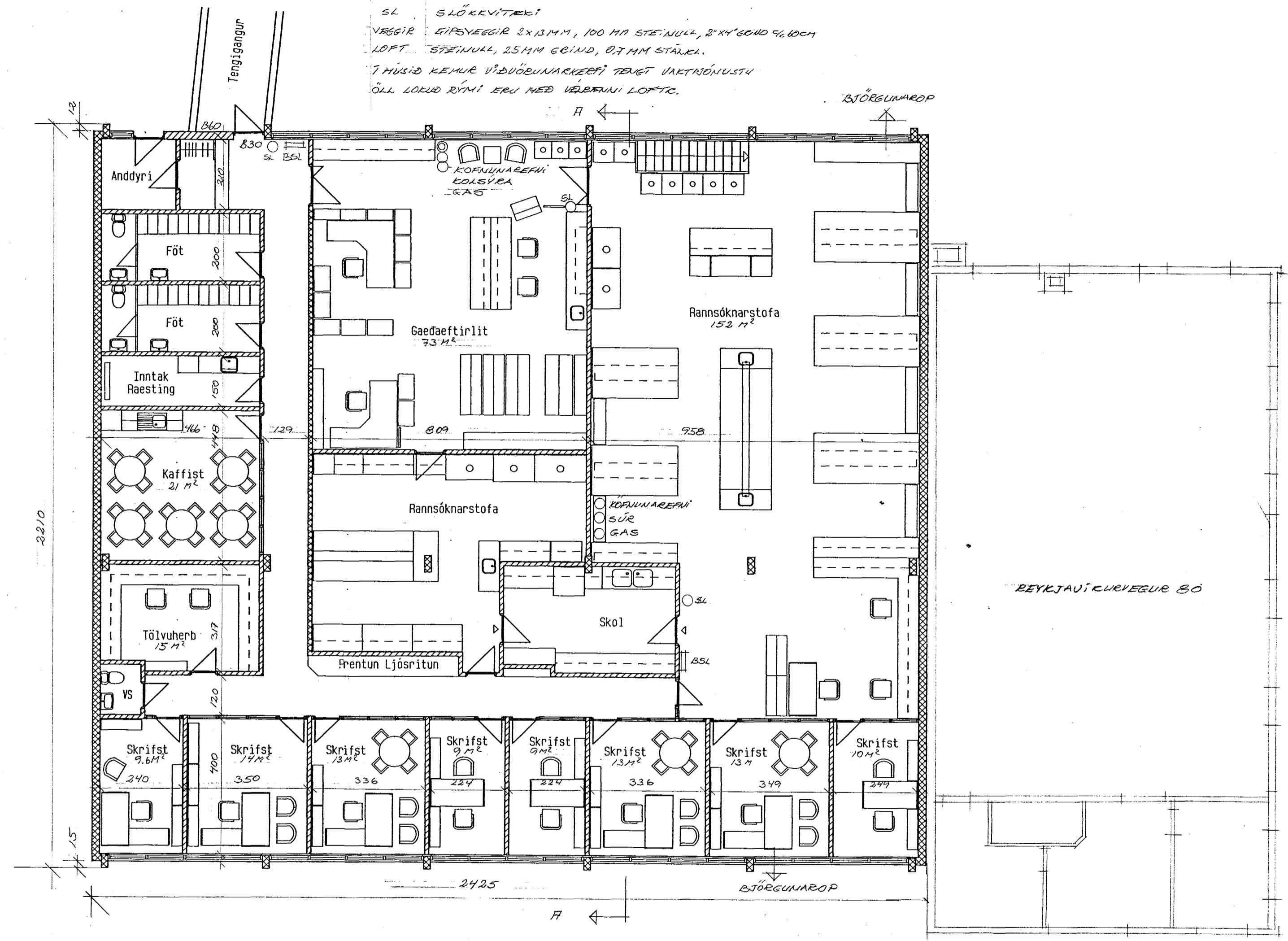
GRUNNMYND 1. HEDAR MKV=1:100
