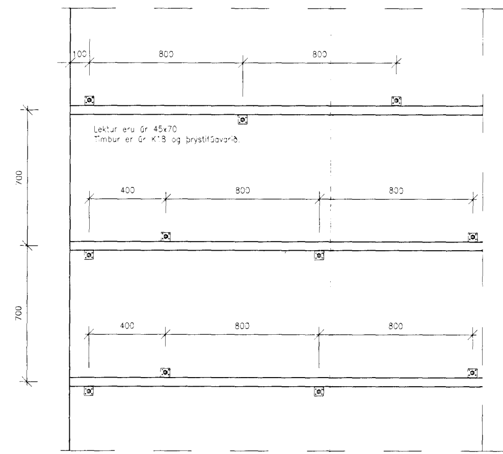
Festing klæðningar á úttegg Ásýnd á úttegg. M 1:10
