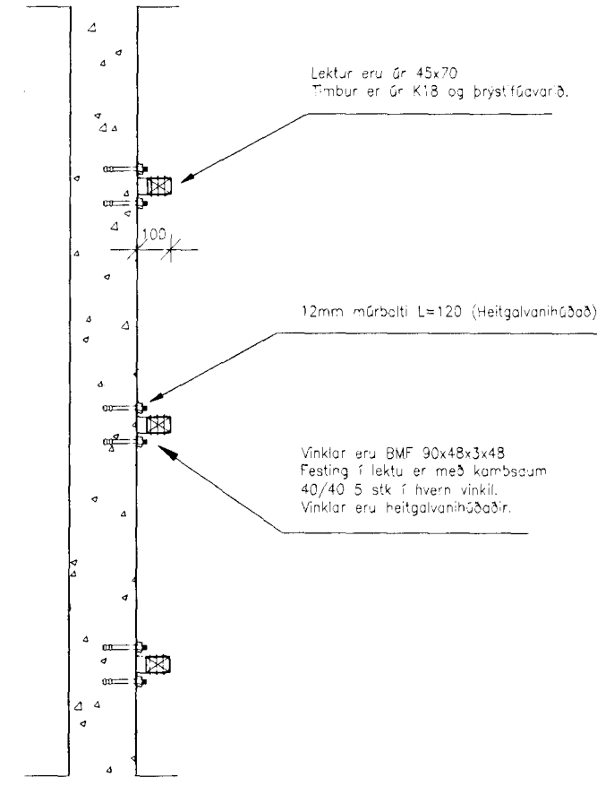
Festing klæðningar á úttegg Hliðarmynd. M 1:10
