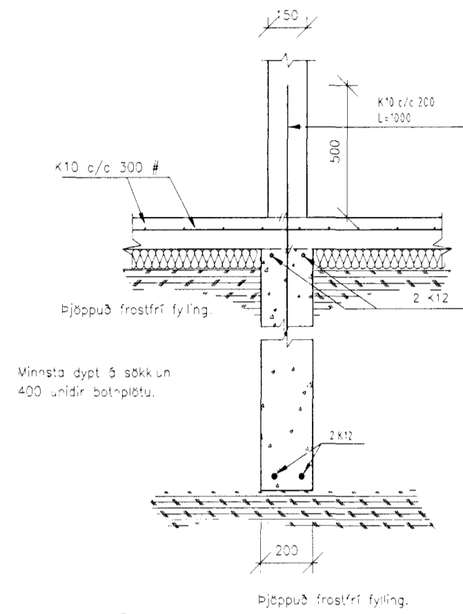
C SNID 871 973 M. 1: 20 Ölfræn frastífrí fylling
