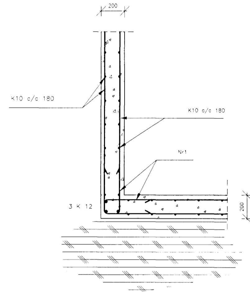
A SNID 871 973 M. 1: 20 Ölfræn bjáppaub frastífrí fylling
