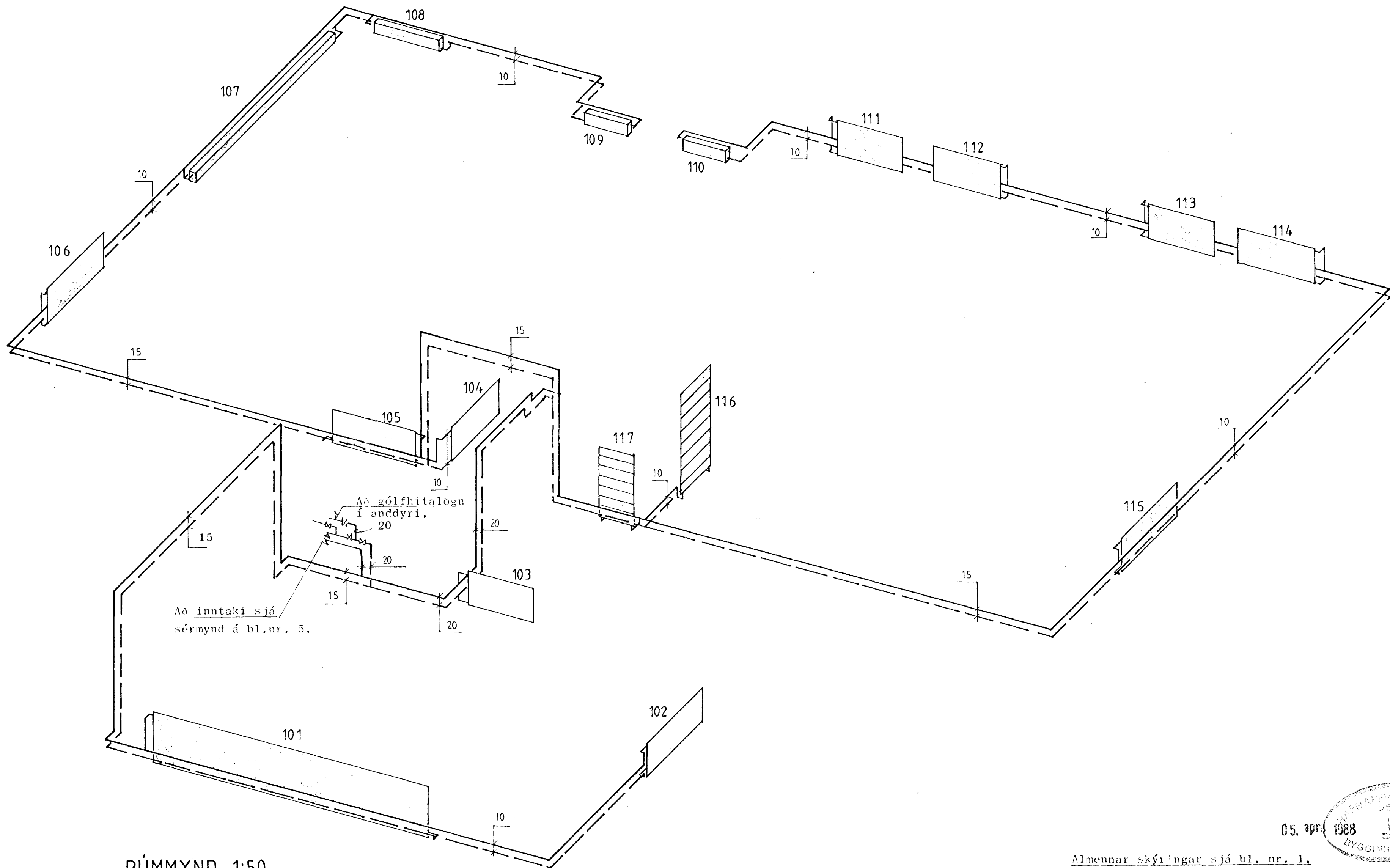
RÚMMYND 1:50
