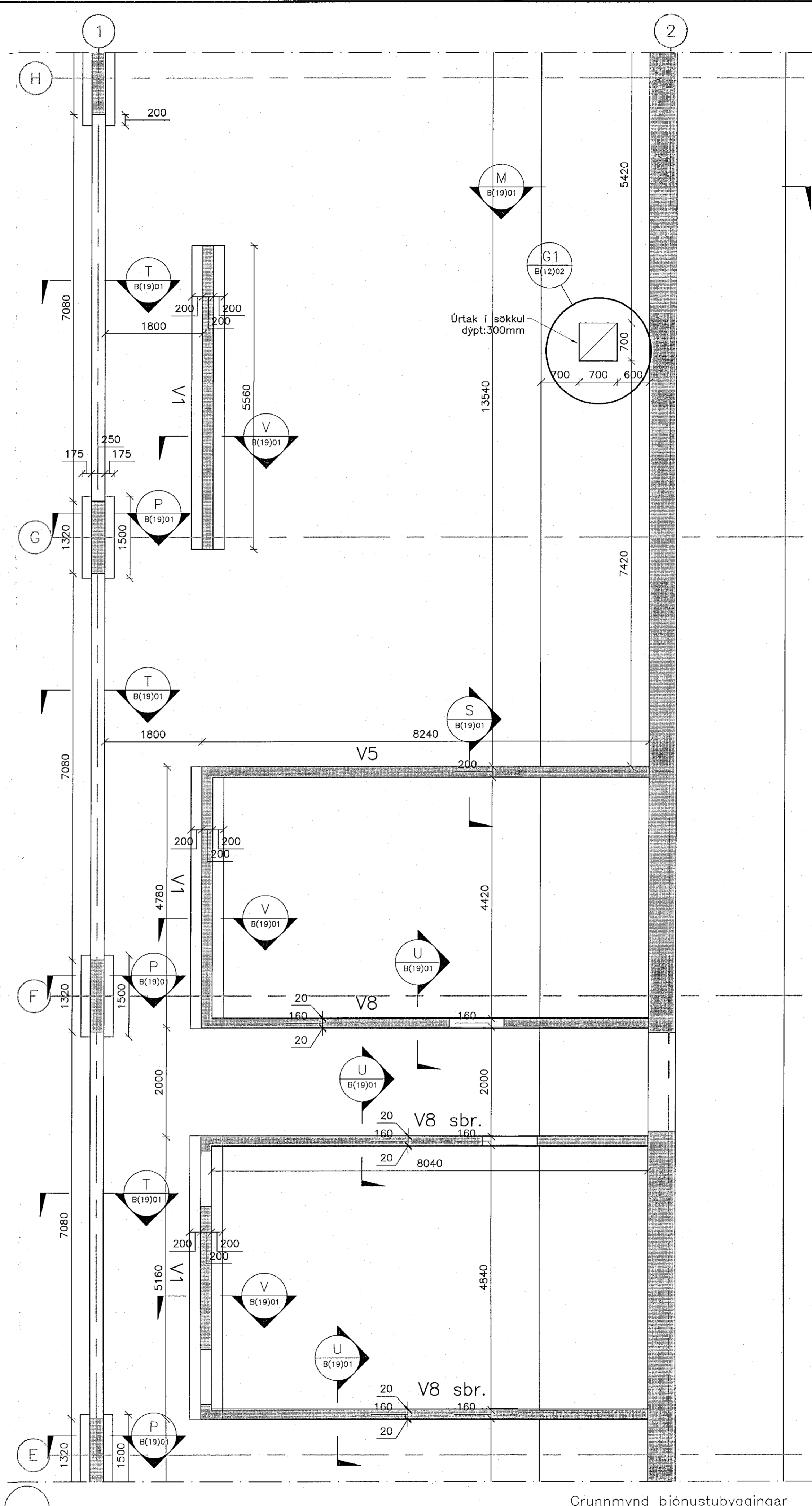
Grunnmynd þjónustubyggingar Mkv: 1:50
