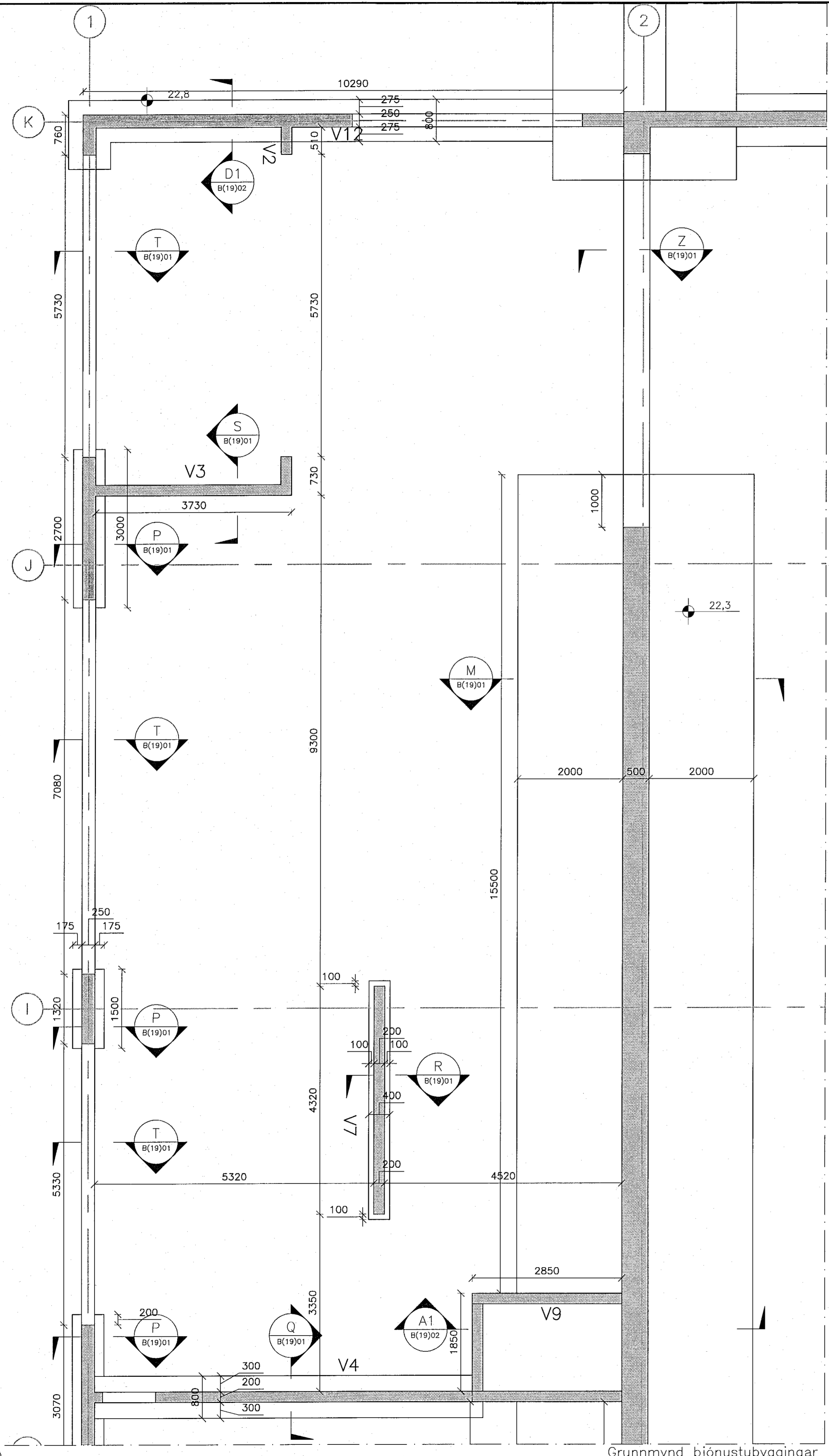
Grunnmynd þjónustubyggingar Mkv: 1:50
