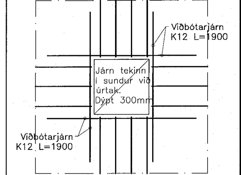
G1 Úrtak i sökkul Mkv: 1:30
