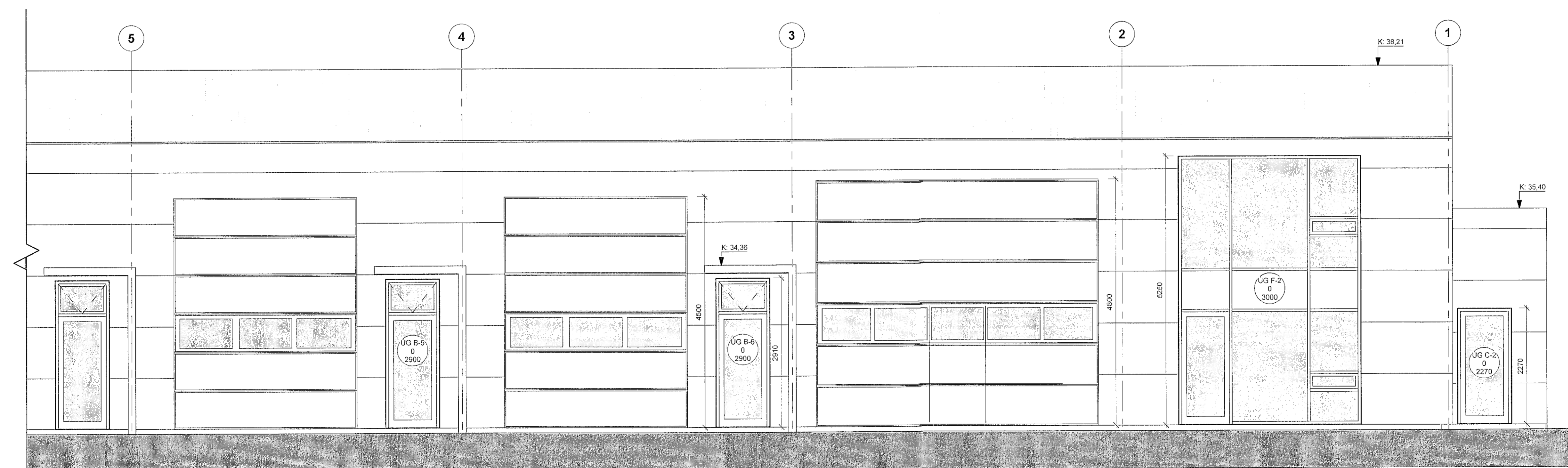
Ásýnd vestur suðurhluti 1 : 50
