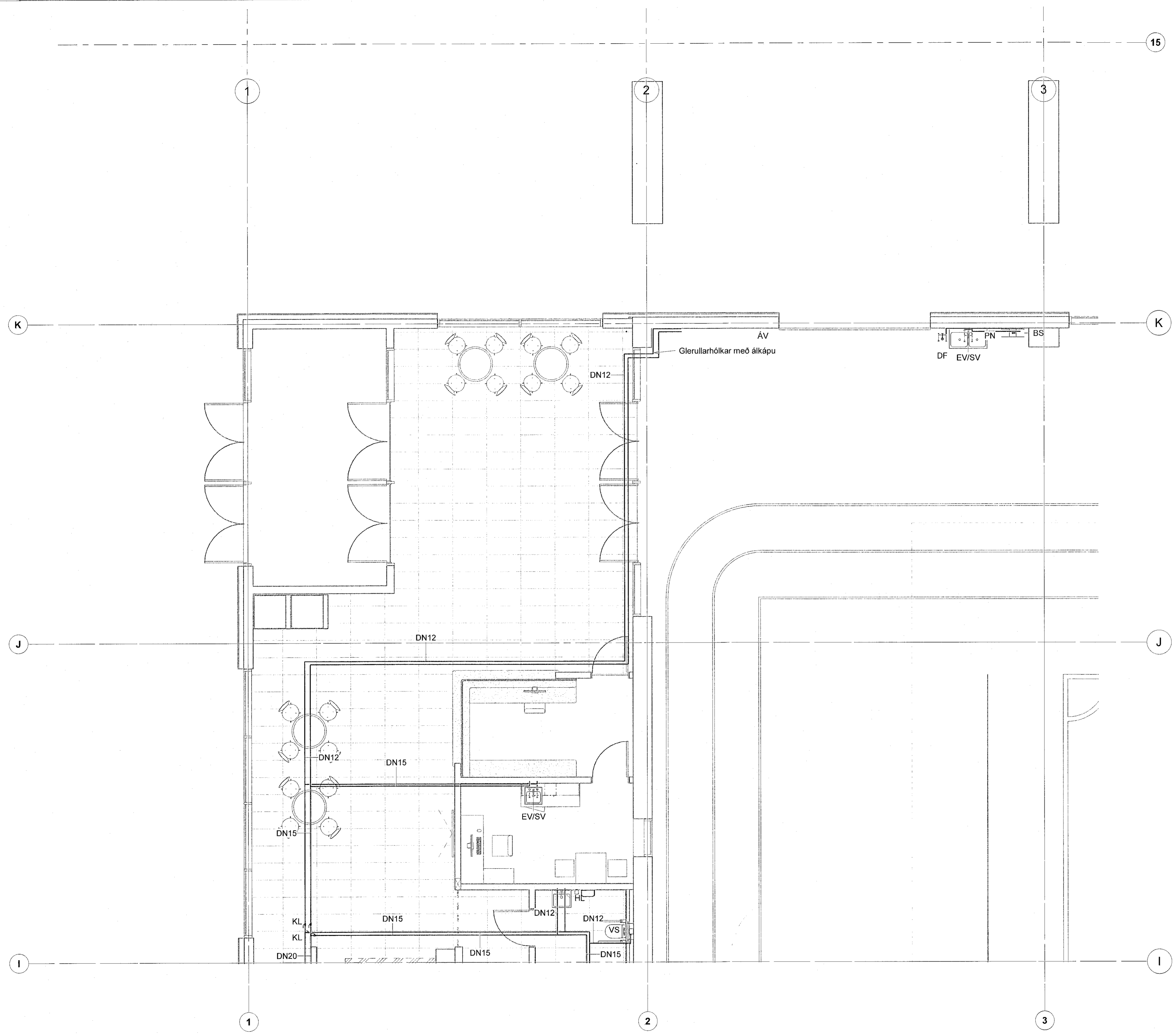
1 Grunnmynd, 1. hæð 1:50
