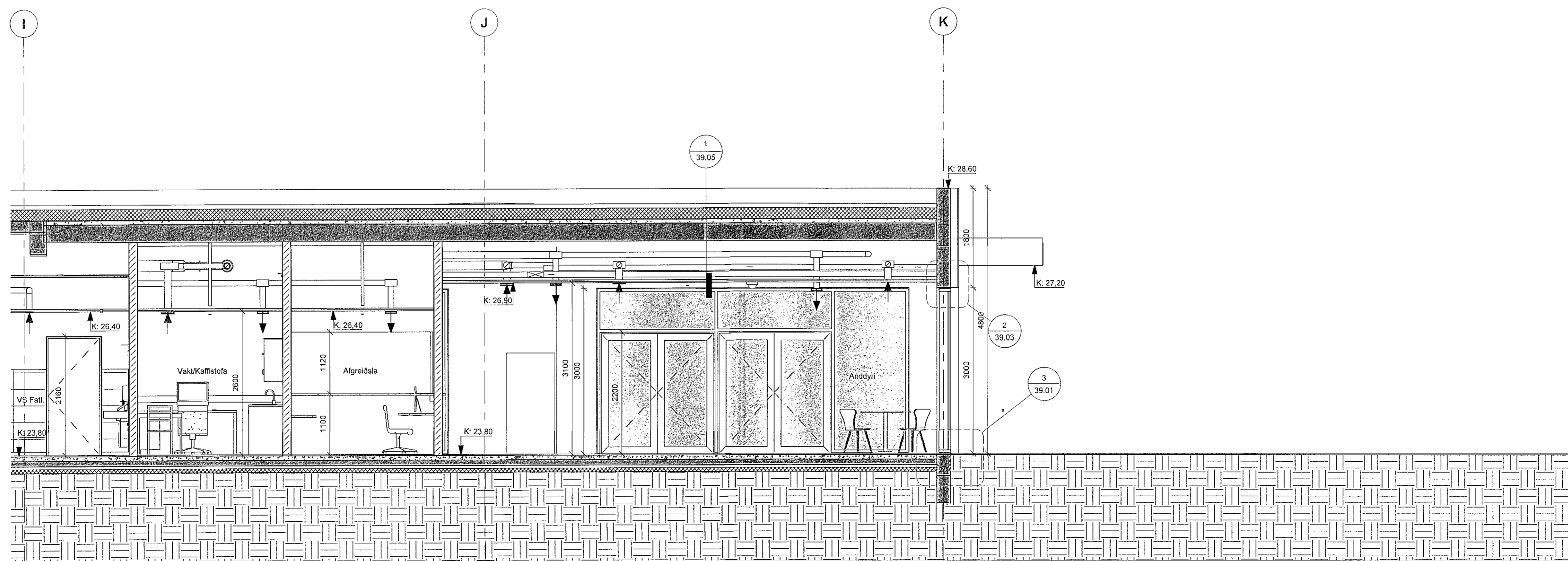
2 20-2-S - Hluti 4 1:50
