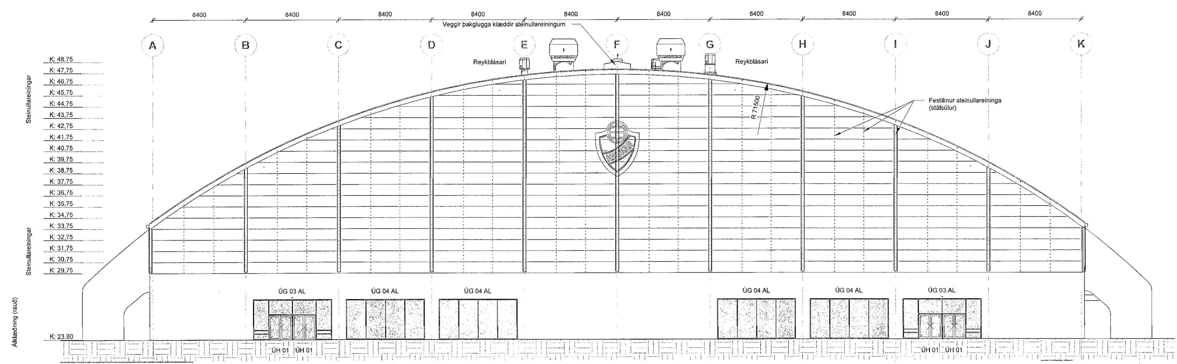
1 Norður - Útlit 1 : 200
