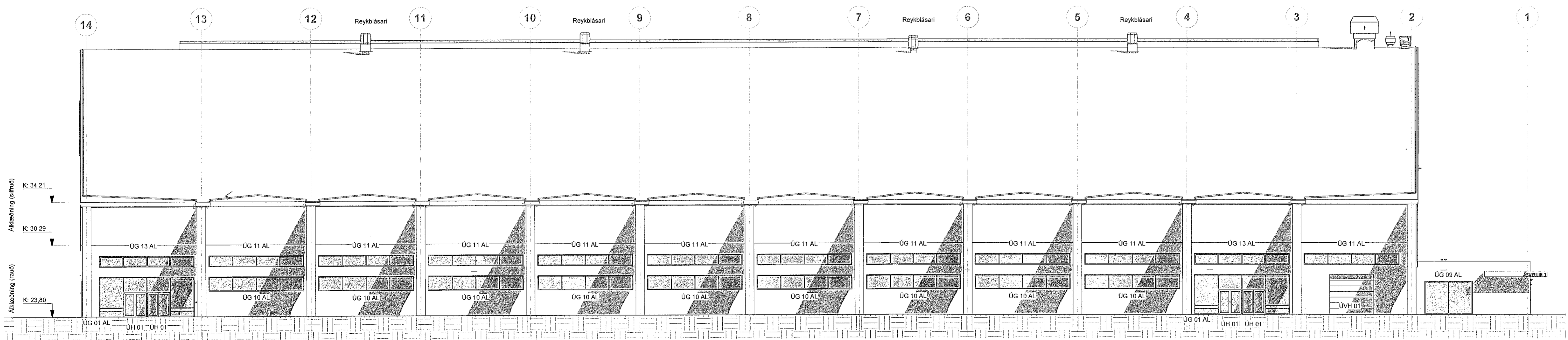
2 Vestur - Útlit 1 : 200
