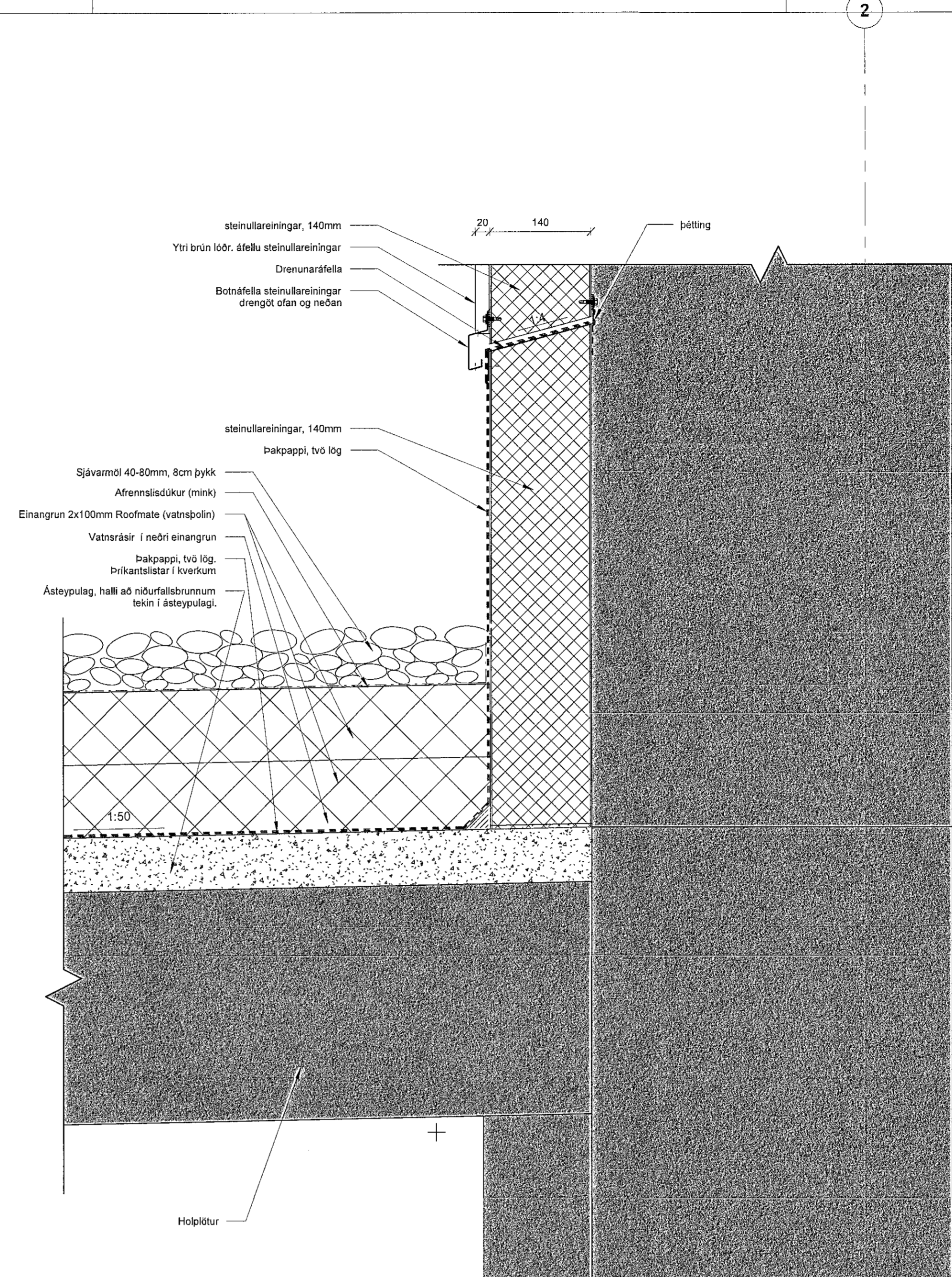
2 Viðsnúid þak, efri, holplötur 1:5
