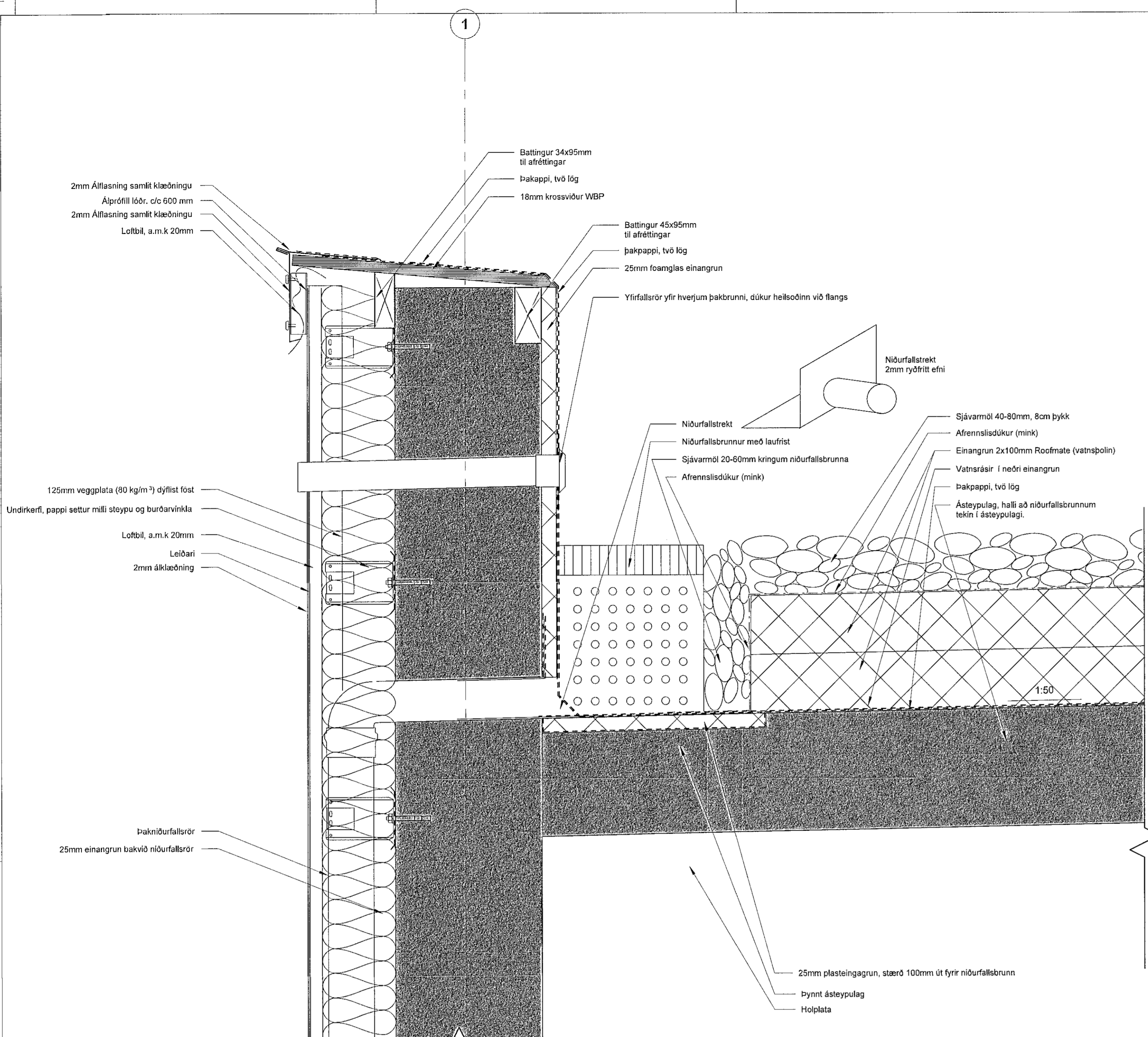
1 Viðsnúid þak, þakbrunnur 1:5
