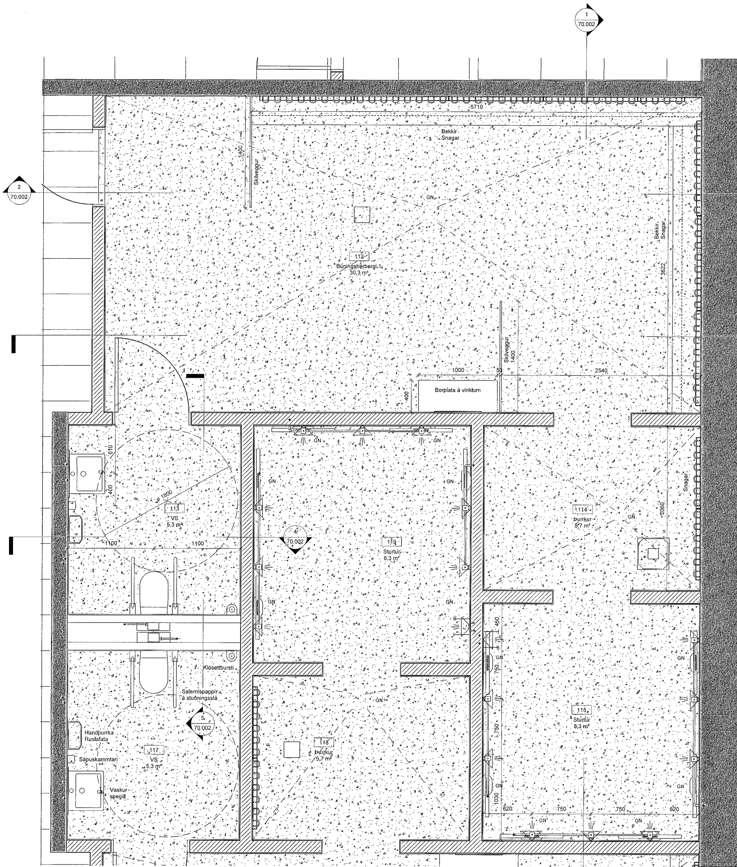
1 Búningsherbergi, þurrkur, sturtur og VS 1 : 25
