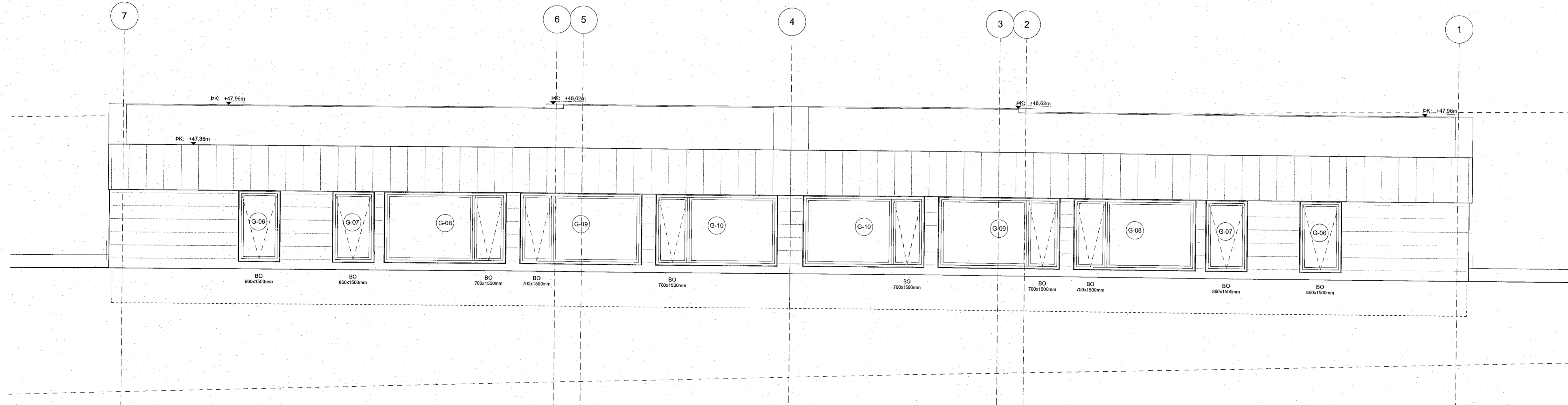
Ásýnd austur mkv: 1:50
