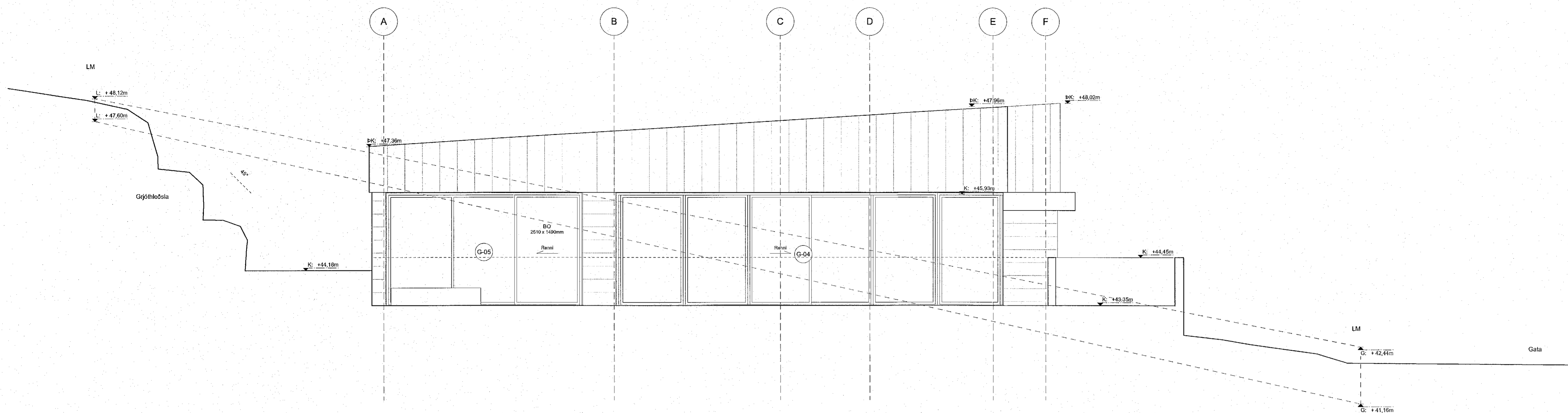
Ásýnd norður mkv: 1:50
