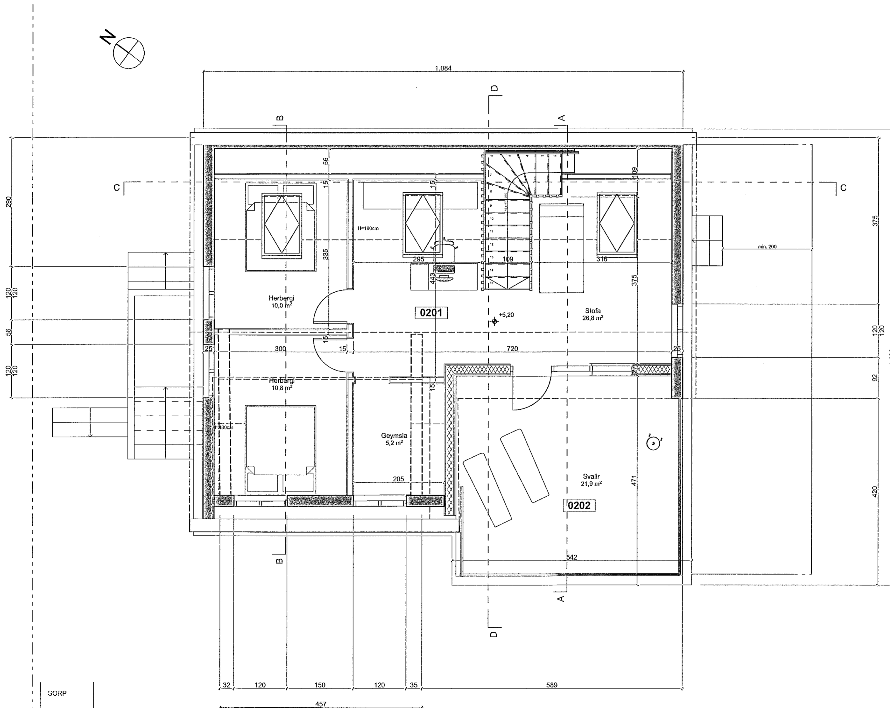
Grunnmynd 2. hæð
