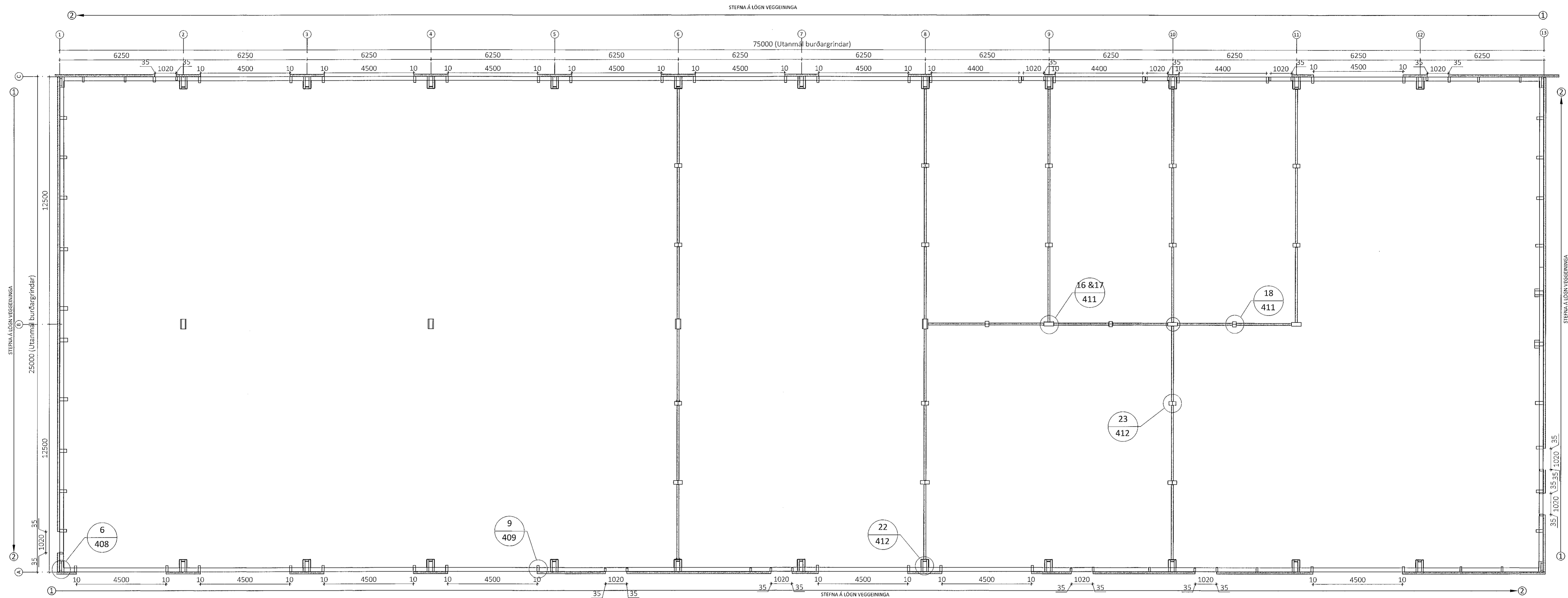
Grunnmynd - Mkv. 1:100
