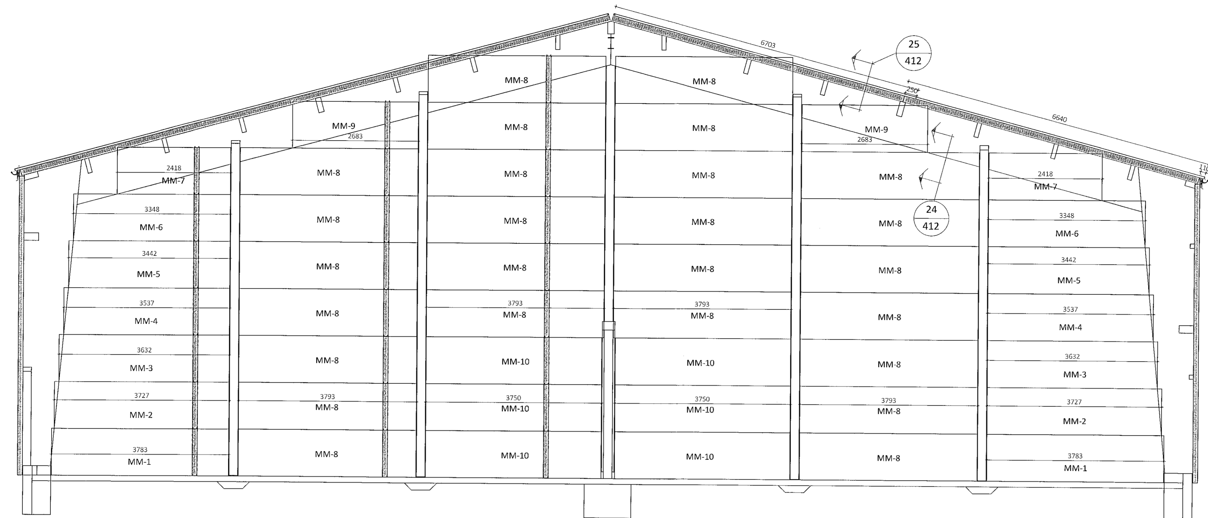
Milliveggur í modu línu 9,10 og 11 mkv 1:50
