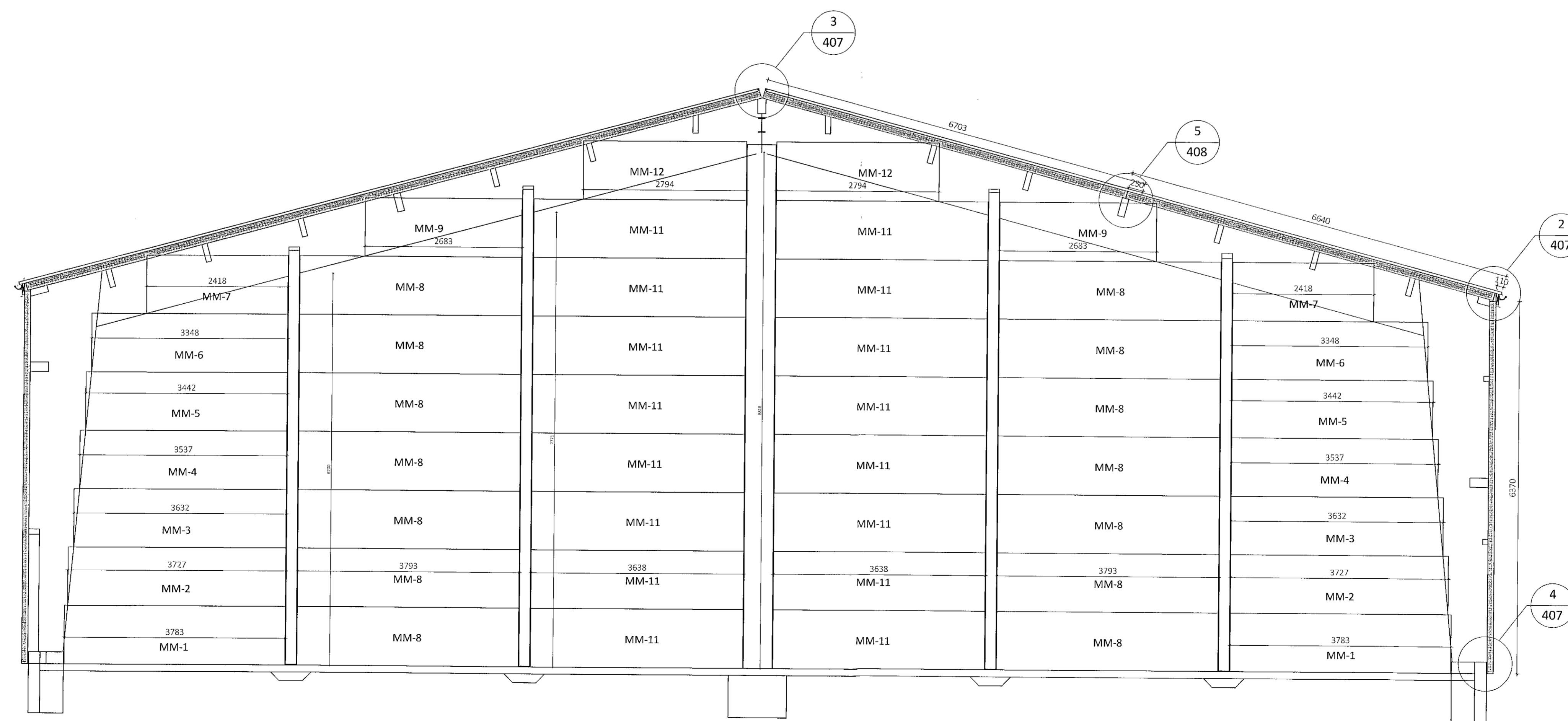
Milliveggur í modu línu 6 og 8 mkv 1:50
