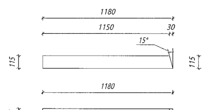
Nr. 142 HB Hurðabiti
