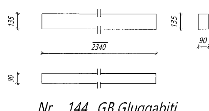
Nr. 144 GB Gluggabiti
