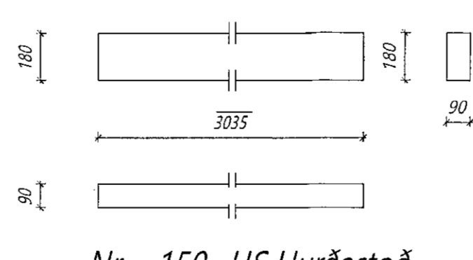
Nr. 150 HS Hurðastoð
