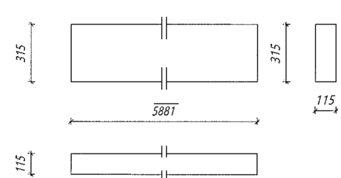
Nr. 141 HS Hurðastoð
