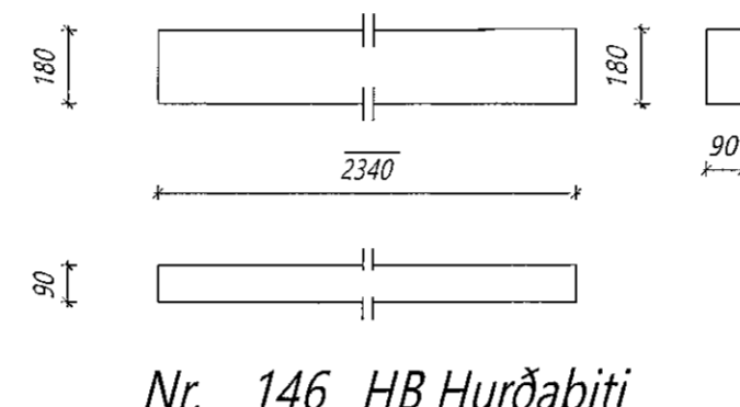
Nr. 146 HB Hurðabiti
