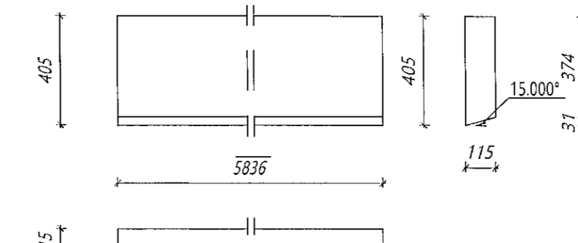
Nr. 152 KB Kantbiti
