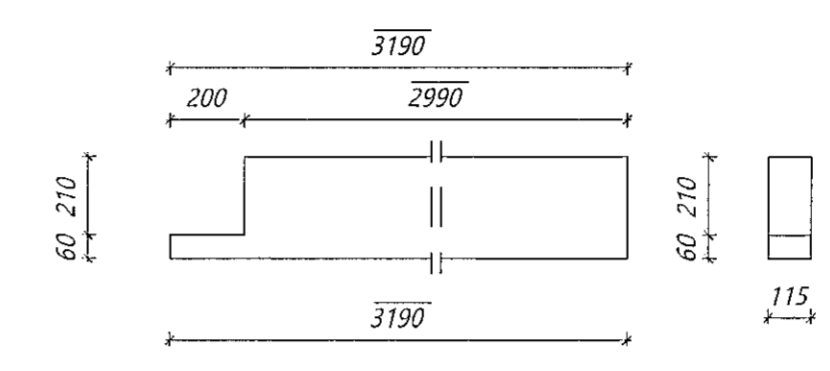
Nr. 178 HS Hurðastoð
