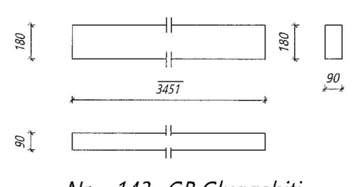
Nr. 143 GB Gluggabiti
