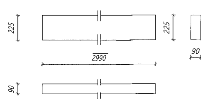
Nr. 149 GLS Gluggastoð
