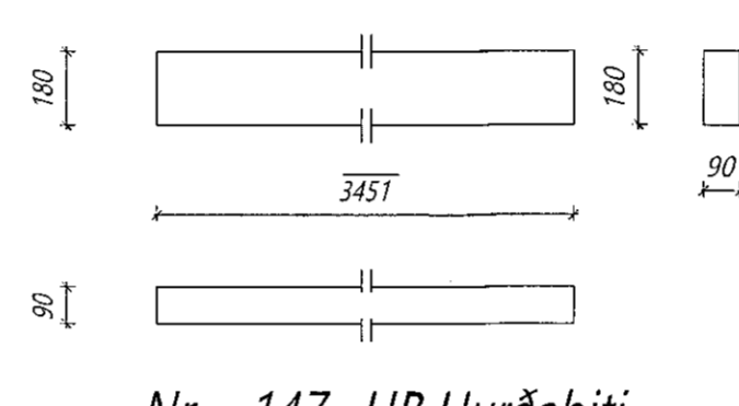
Nr. 147 HB Hurðabiti
