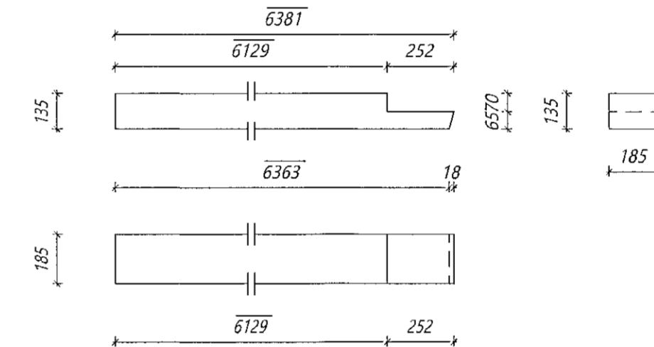
Nr. 224 MS Milliveggir stoð Límré: 185*135, L=6381 mm Samtals: 6 stk.
