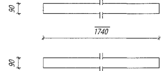
Nr. 221 VB Veggbiti langhlið Límré: 90*90, L=1740 mm Samtals: 2 stk.
