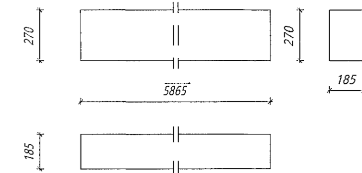
Nr. 199 MV Milliveggur þverbiti Límré: 185*270, L=5865 mm Samtals: 1 stk.
