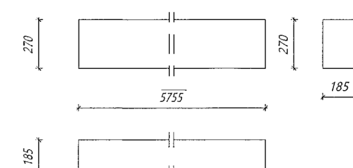
Nr. 200 MV Milliveggur þverbiti Límré: 185*270, L=5755 mm Samtals: 2 stk.
