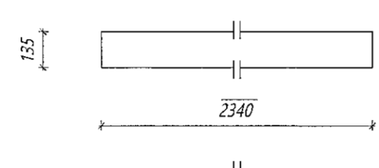
Nr. 222 VB Veggbiti langhlið Límré: 90*135, L=2340 mm Samtals: 4 stk.
