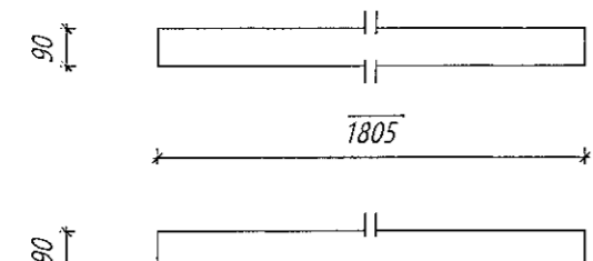
Nr. 215 VB Veggbiti langhlið Límré: 90*90, L=1805 mm Samtals: 1 stk.
