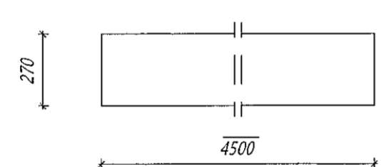
Nr. 219 HB Hurðabiti Límré: 115*270, L=4500 mm Samtals: 1 stk.
