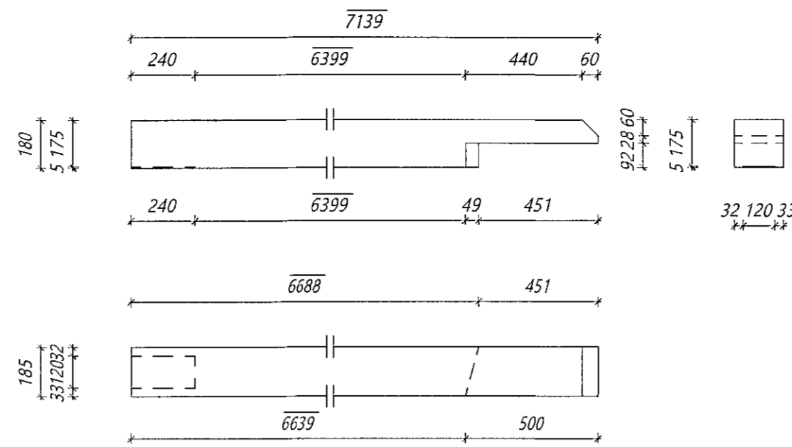
Nr. 195 MS Milliveggir stoð Límré: 185*180, L=7139 mm Samtals: 8 stk.
