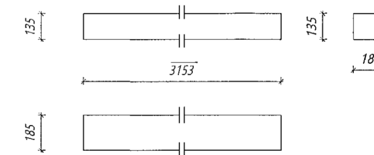
Nr. 225 MS Milliveggir stoð Límré: 185*135, L=3153 mm Samtals: 6 stk.
