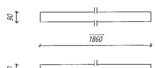
Nr. 213 VB Veggbiti langhlið Límré: 90*90, L=1860 mm Samtals: 9 stk.
