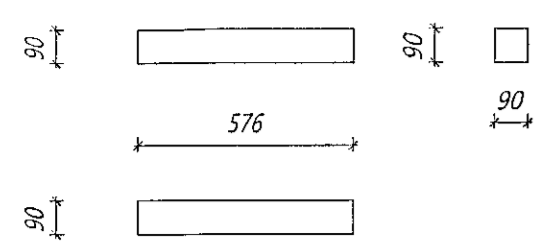
Nr. 210 VB Veggbiti langhlið Límré: 90*90, L=576 mm Samtals: 27 stk.
