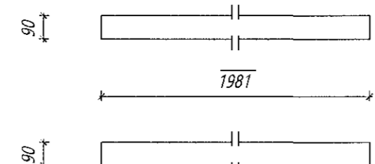
Nr. 220 VB Veggbiti langhlið Límré: 90*90, L=1981 mm Samtals: 1 stk.
