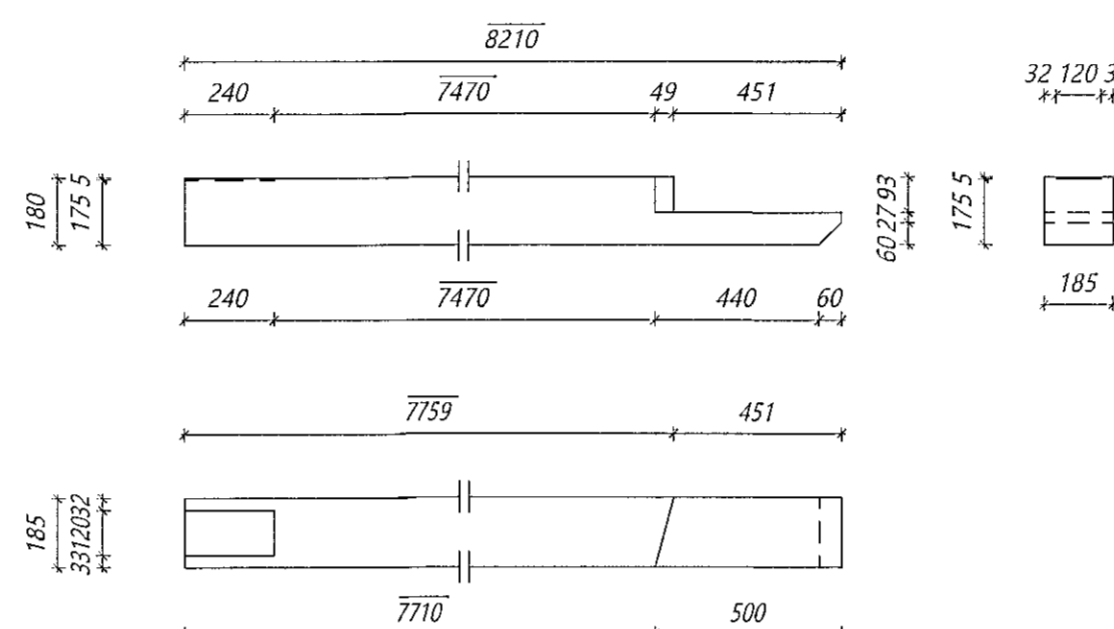
Nr. 196 MS Milliveggir stoð Límré: 185*180, L=8210 mm Samtals: 8 stk.
