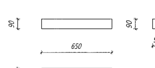
Nr. 223 GB Gluggabiti Límré: 90*90, L=650 mm Samtals: 1 stk.
