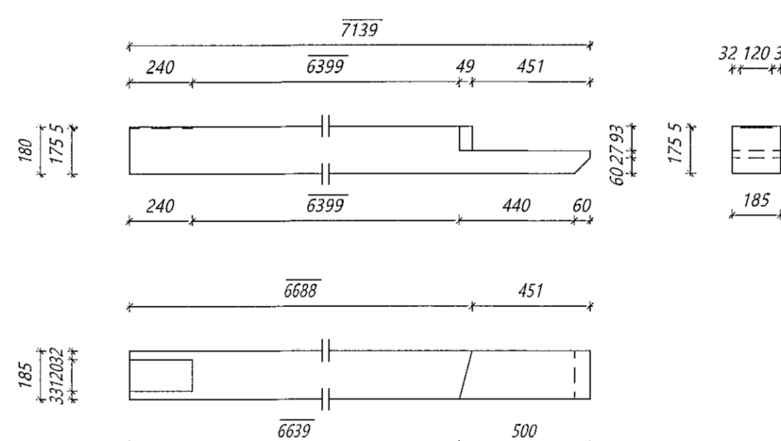
Nr. 197 MS Milliveggir stoð Límré: 185*180, L=7139 mm Samtals: 8 stk.
