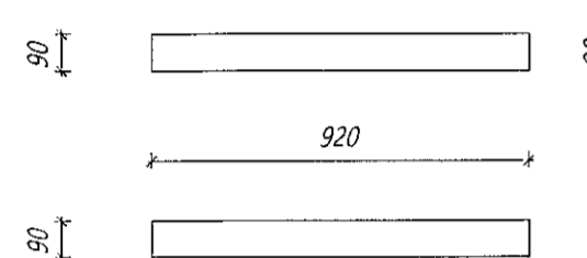
Nr. 212 VB Veggbiti langhlið Límré: 90*90, L=920 mm Samtals: 2 stk.
