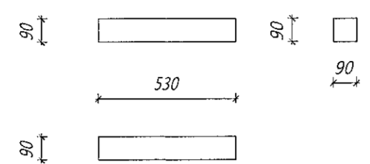
Nr. 216 VB Veggbiti langhlið Límré: 90*90, L=530 mm Samtals: 1 stk.
