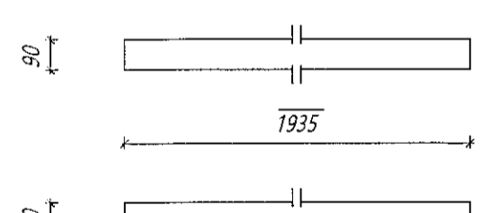
Nr. 214 VB Veggbiti langhlið Límré: 90*90, L=1935 mm Samtals: 5 stk.
