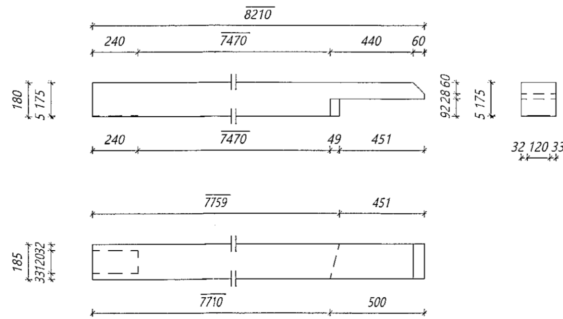
Nr. 198 MS Milliveggir stoð Límré: 185*180, L=8210 mm Samtals: 8 stk.
