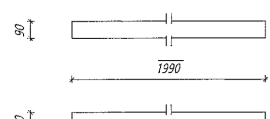
Nr. 218 VB Veggbiti langhlið Límré: 90*90, L=1990 mm Samtals: 1 stk.
