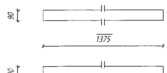
Nr. 211 VB Veggbiti langhlið Límré: 90*90, L=1375 mm Samtals: 2 stk.
