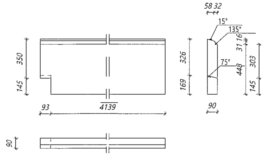
Nr. 237 PG Þakgluggi Límré: 90*495, L=4232 mm Samtals: 1 stk.
