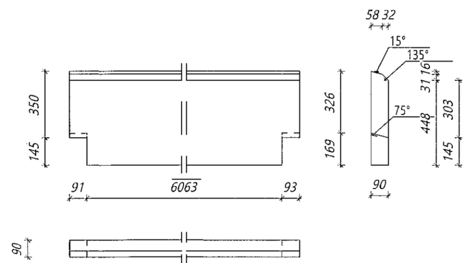
Nr. 235 PG Þakgluggi Límré: 90*495, L=6247 mm Samtals: 1 stk.
