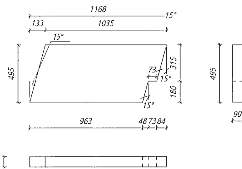
Nr. 228 PG Þakgluggi Límré: 90*495, L=1168 mm Samtals: 4 stk.
