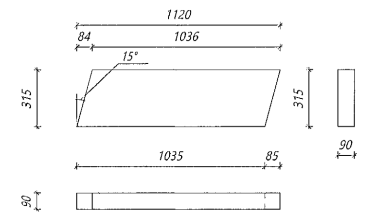
Nr. 231 PG Þakgluggi Límré: 90*315, L=1120 mm Samtals: 2 stk.
