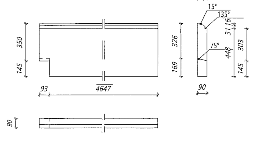
Nr. 241 PG Þakgluggi Límré: 90*495, L=4740 mm Samtals: 2 stk.
