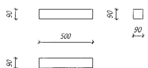
Nr. 125 HB Hurðabiti Límré: 90*90, L=500 mm Samtals: 32 stk.
