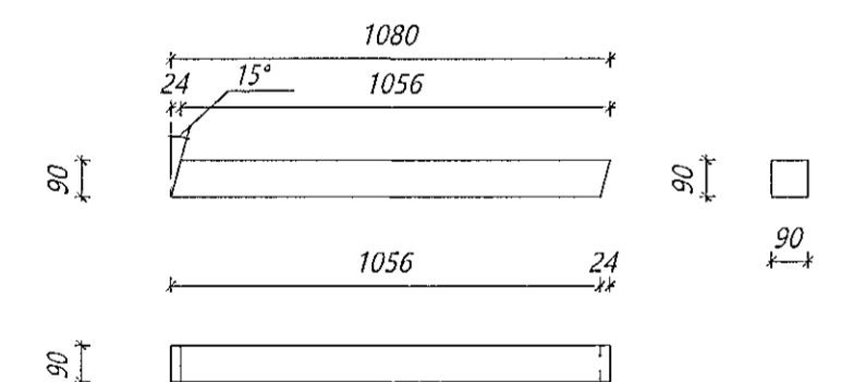
Nr. 232 PG Þakgluggi Límré: 90*90, L=1080 mm Samtals: 4 stk.
