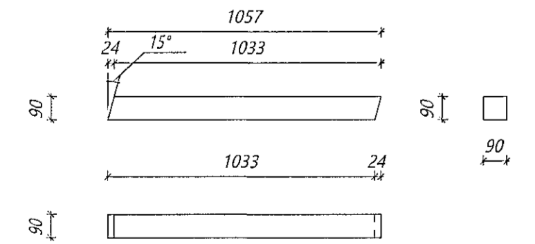
Nr. 233 PG Þakgluggi Límré: 90*90, L=1057 mm Samtals: 10 stk.
