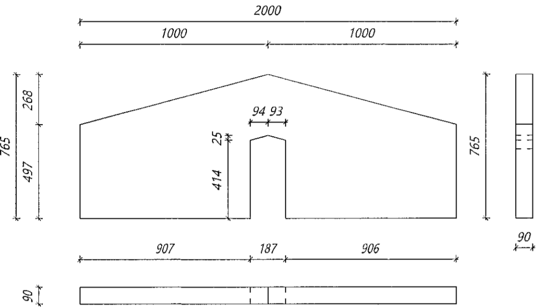
Nr. 230 PG Þakgluggi Límré: 90*765, L=2000 mm Samtals: 5 stk.
