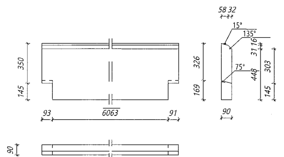
Nr. 234 PG Þakgluggi Límré: 90*495, L=6247 mm Samtals: 1 stk.
