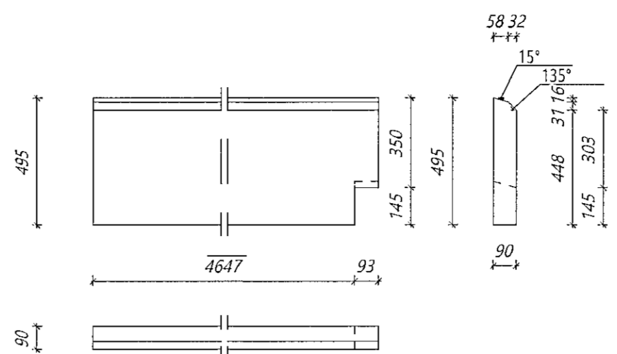
Nr. 242 PG Þakgluggi Límré: 90*495, L=4740 mm Samtals: 2 stk.
