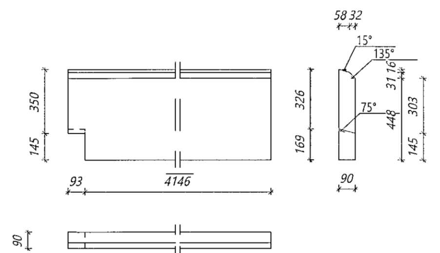
Nr. 239 PG Þakgluggi Límré: 90*495, L=4239 mm Samtals: 4 stk.
