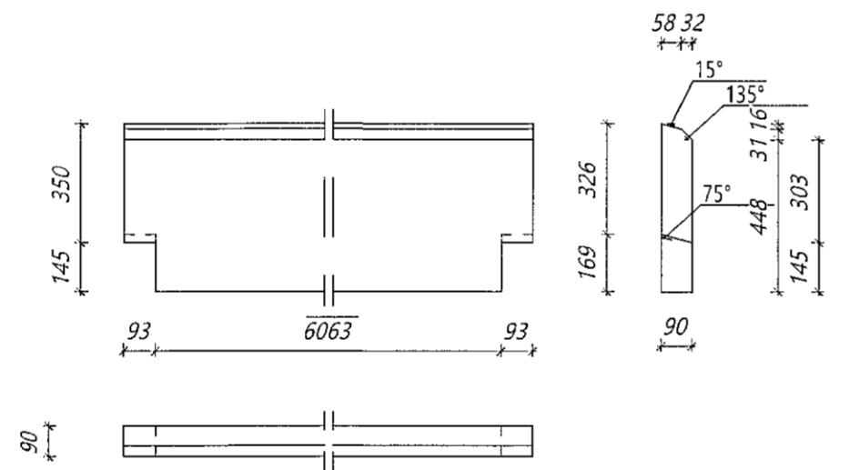
Nr. 236 PG Þakgluggi Límré: 90*495, L=6249 mm Samtals: 4 stk.
