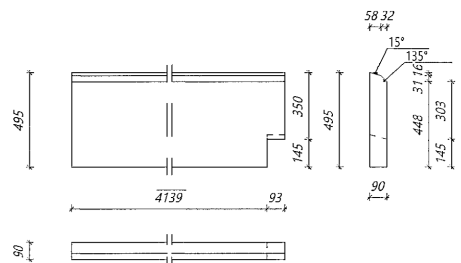
Nr. 238 PG Þakgluggi Límré: 90*495, L=4232 mm Samtals: 1 stk.
