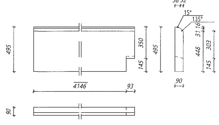
Nr. 240 PG Þakgluggi Límré: 90*495, L=4239 mm Samtals: 4 stk.
