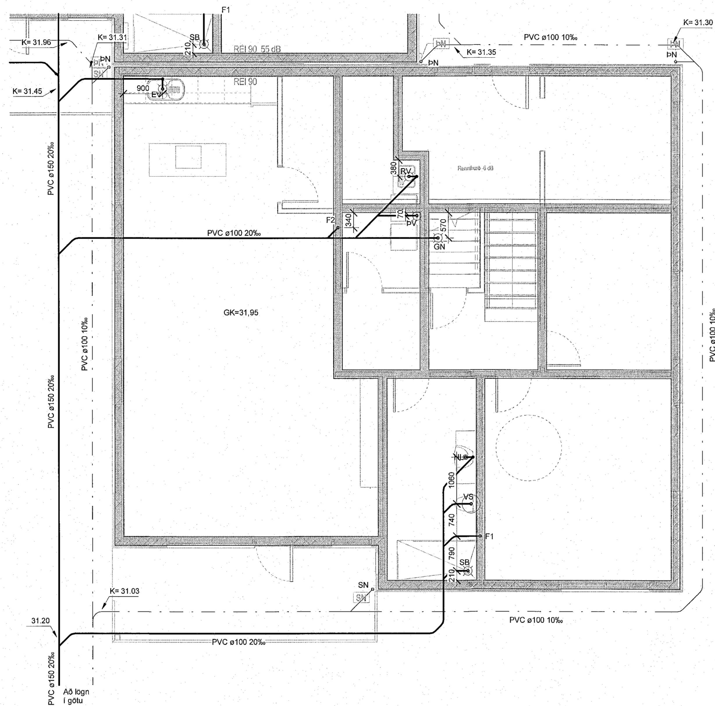
1 1. hæð - Grunnmynd 2 1 : 50
