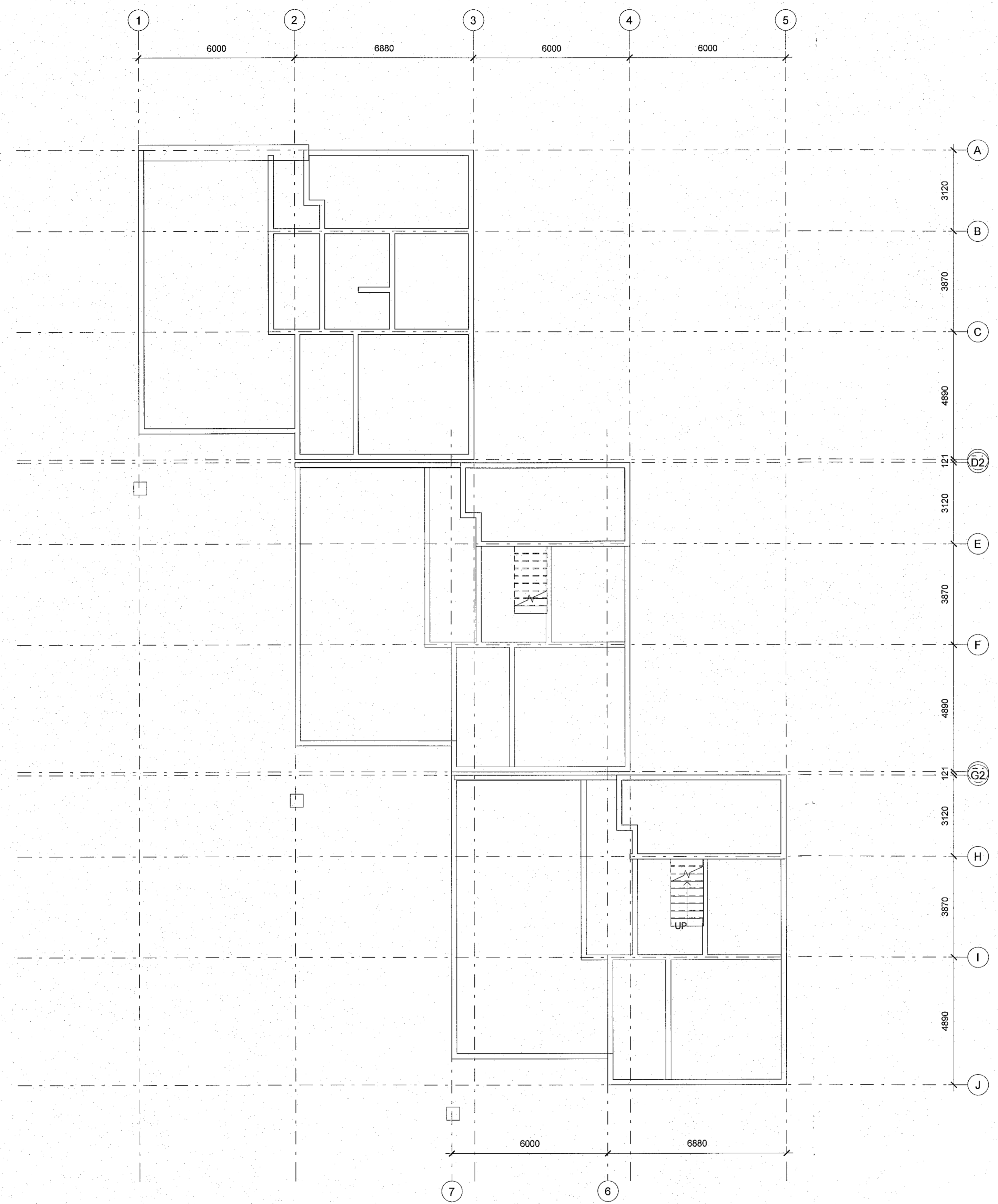
1 000- Undirstöður Yfirlit 1:100
