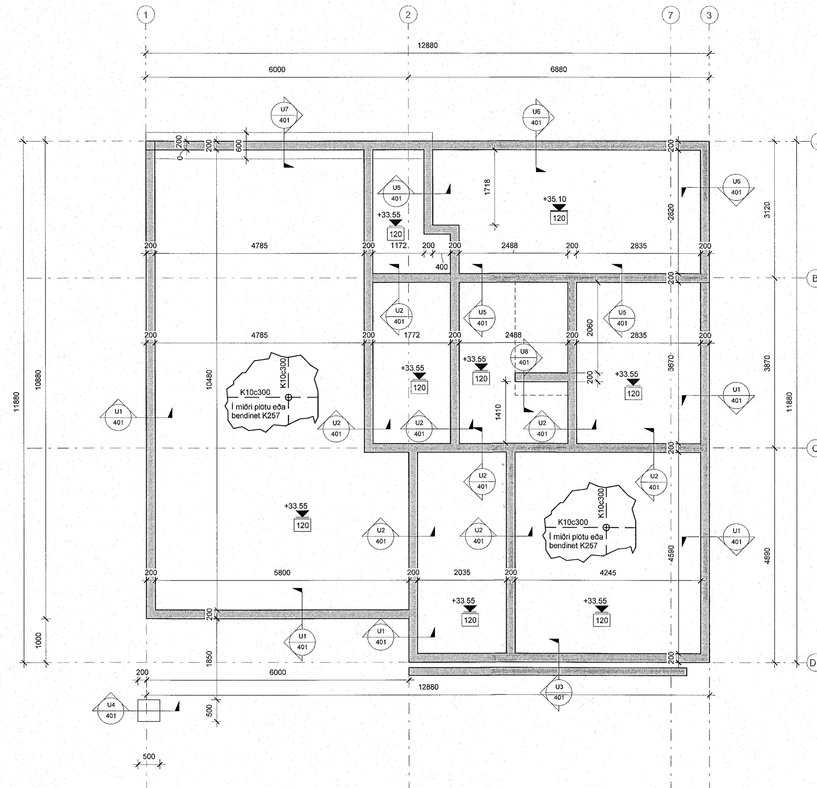
1 001-Undirstöður Hús Nr.2 1:50
