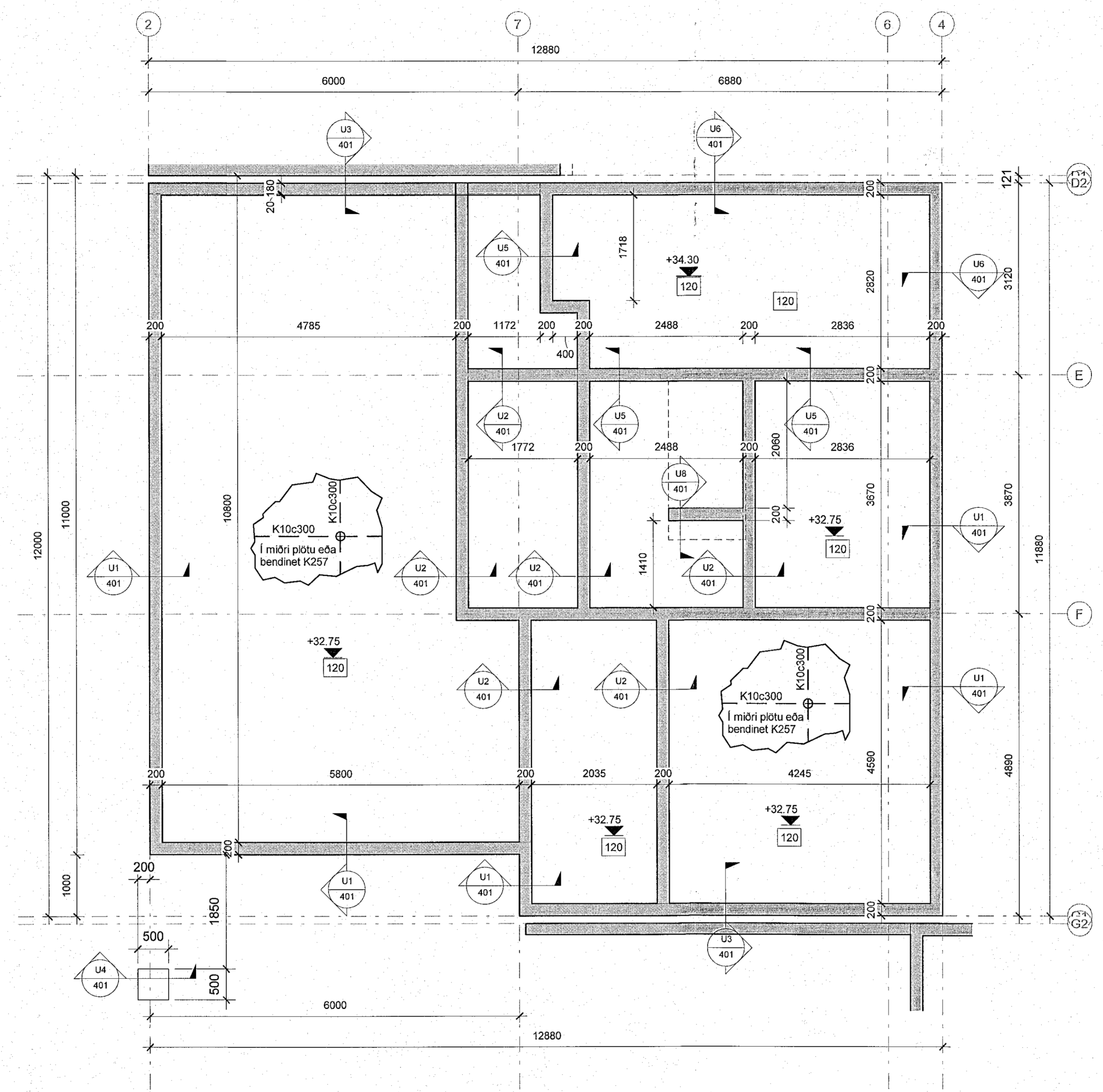
1 002- Undirstöður Hús Nr.4 1 : 50
