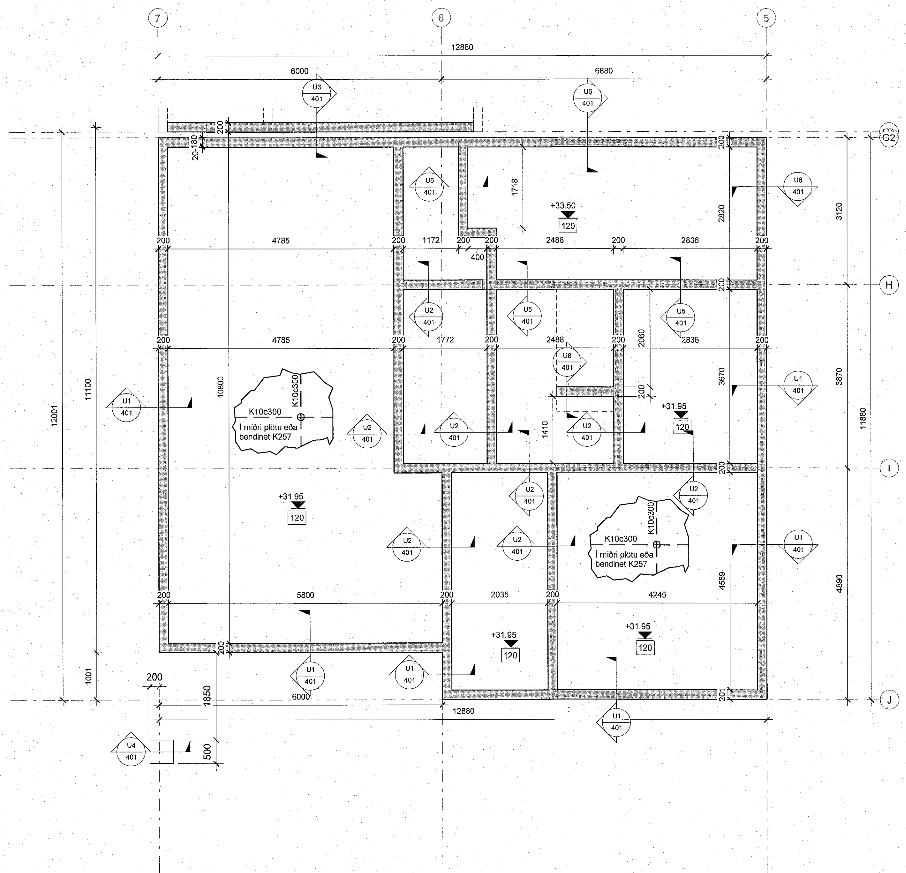
1 003- Undirstöður Hús Nr.6 1 : 50
