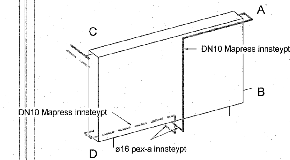
Dæmigerð tenging á ofni séð aftan frá
