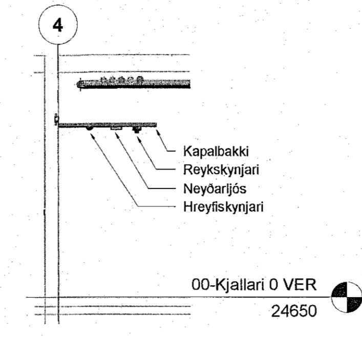
ED Snið ED 00_3_14_01 1 : 50
