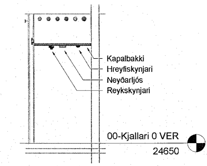
EE Snið EE 00_3_14_01 1 : 50
