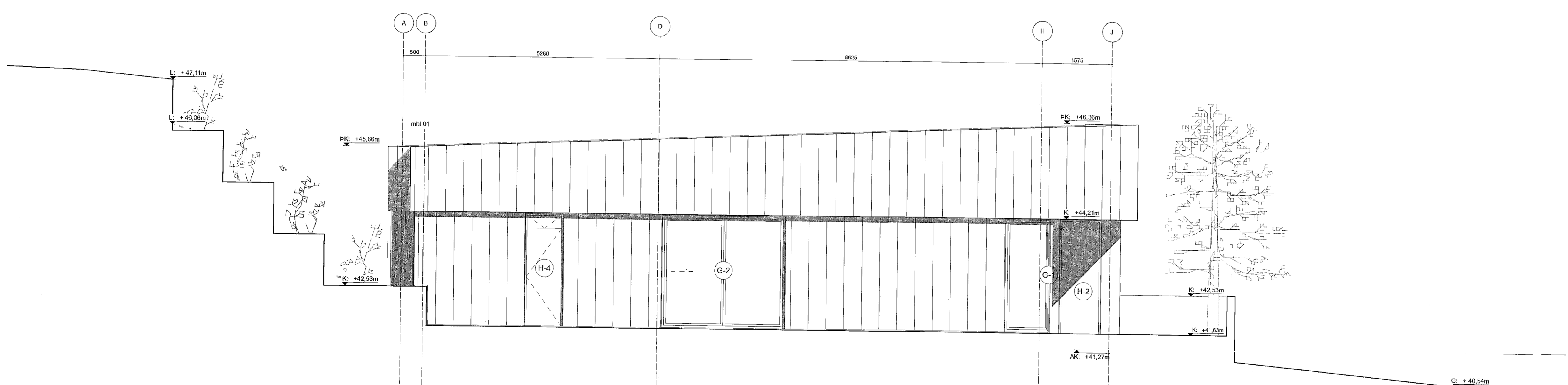
Ásýnd norður mkv: 1:50/1:100
